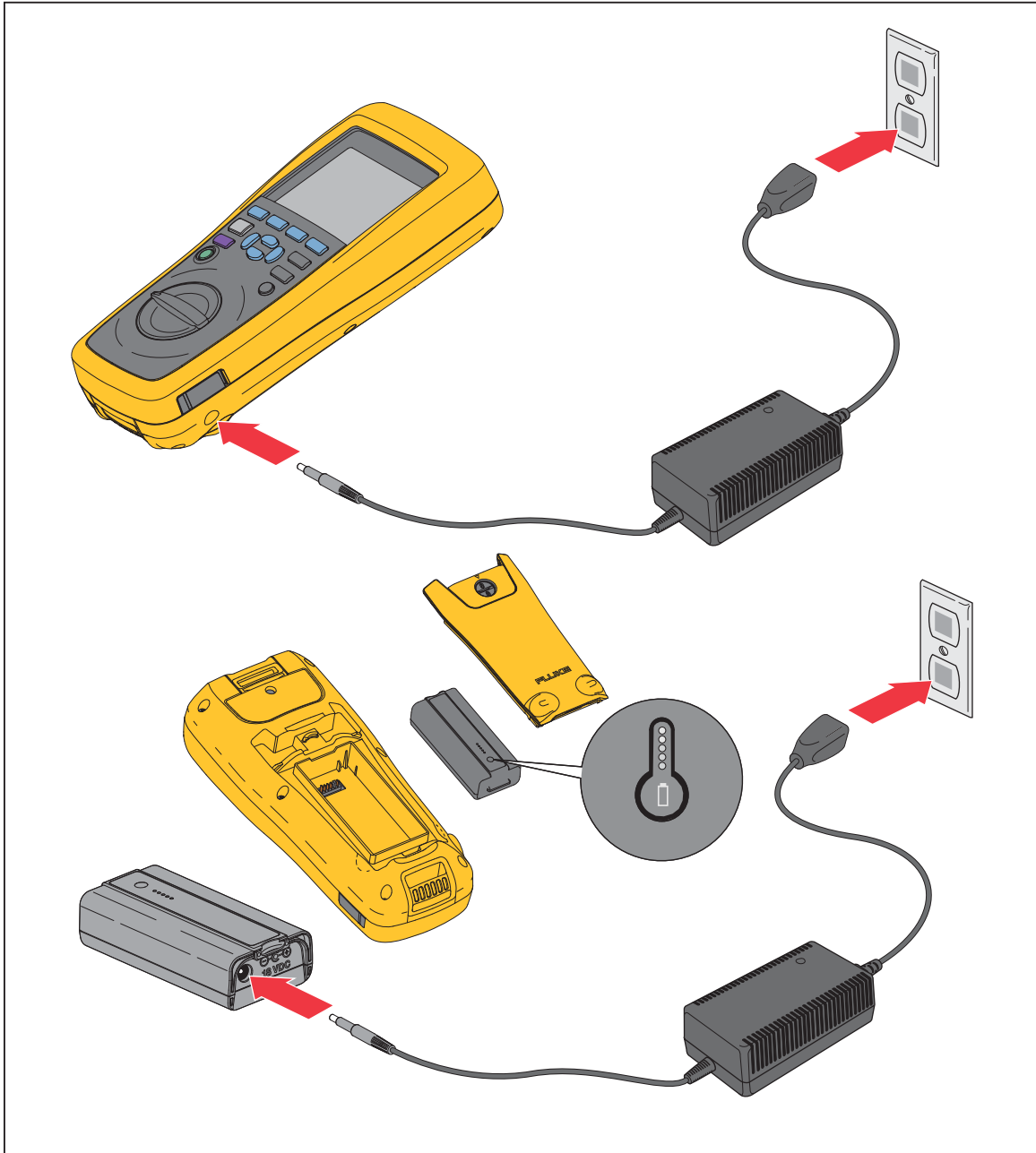
Figura 6-5. Carga de la batería
