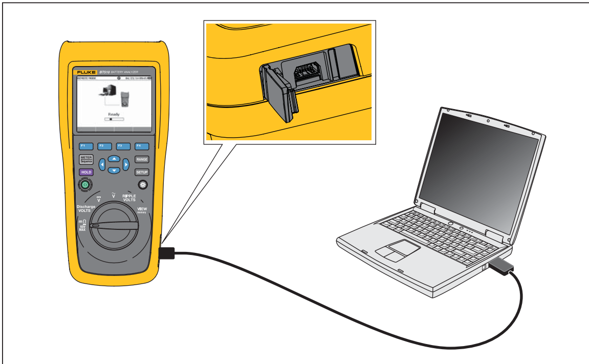
Figura 5-1. Conexión a PC
