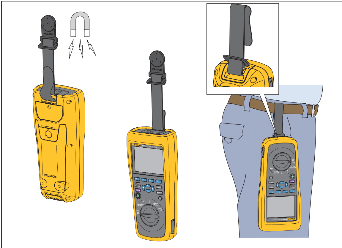
Figura 2-2. Correa para cinturón
