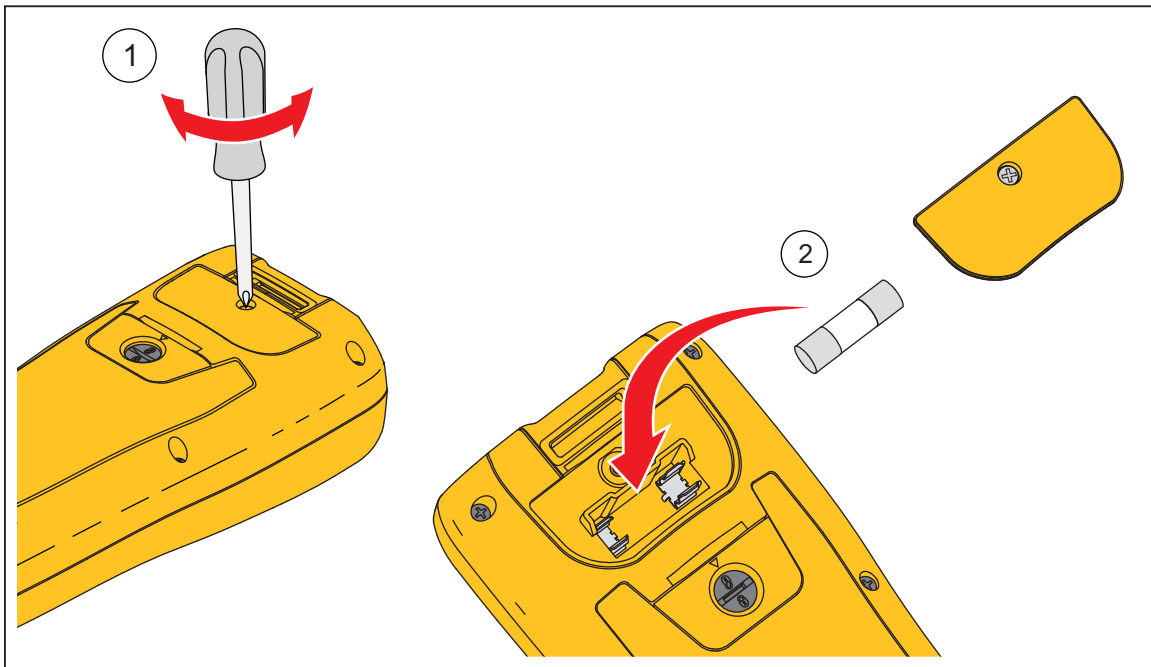
Figura 6-2. Sustitución del fusible
