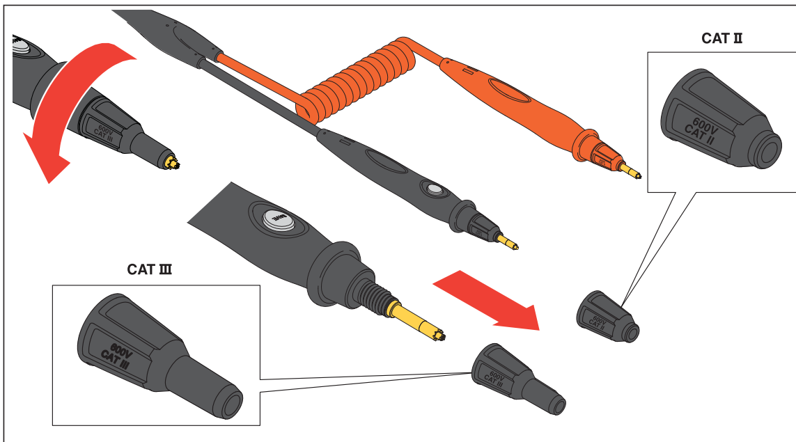
Figura 6-3. Sustitución de las puntas de sonda
