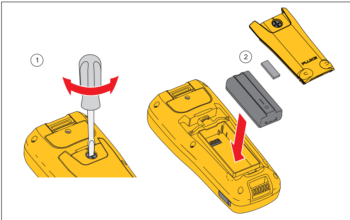
Figura 6-1. Instalación o sustitución de un juego de baterías
