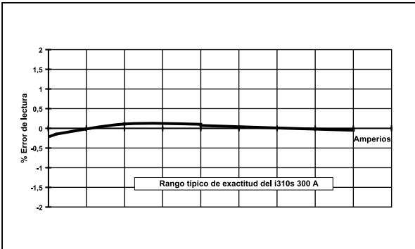
Curva típica de exactitud
