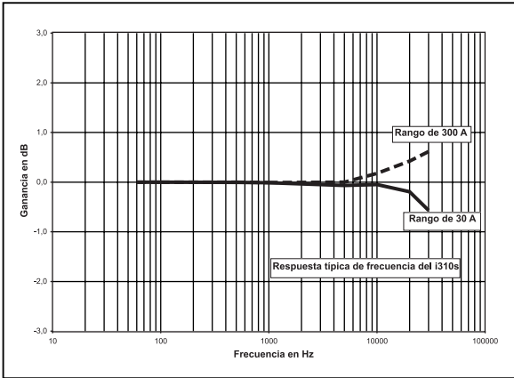
Respuesta típica de frecuencia
