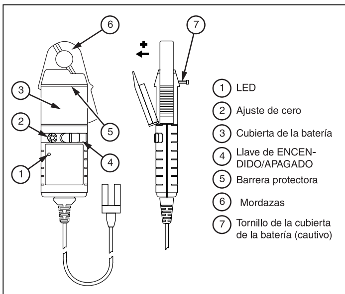
Figura 1. Pinza amperimétrica para CA/CC i310s
