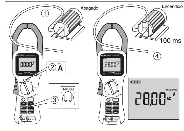
Figura 4. Medición de la corriente de arranque
