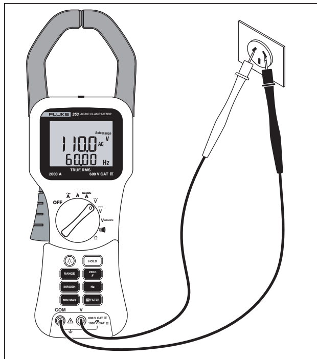
Figura 5. AC Medición de voltaje de CA
