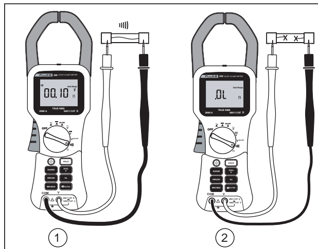
Figura 7. Medición de continuidad
