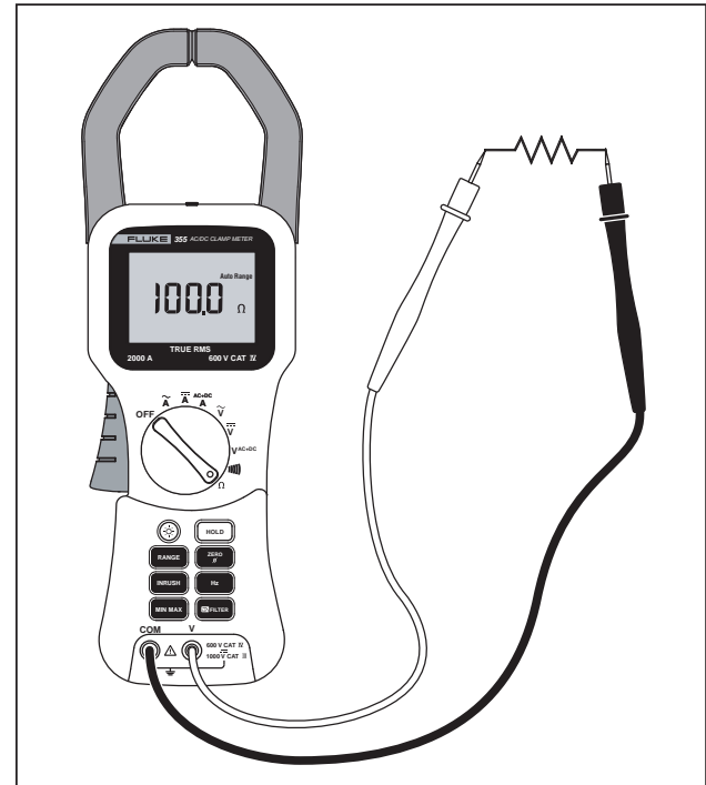
Figura 8. Medición de resistencia
