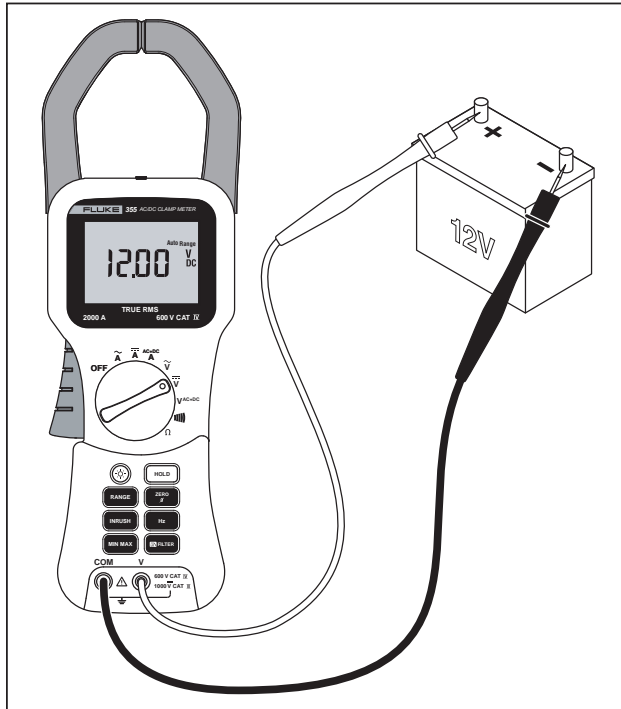
Figura 6. Medición de voltaje de CC
