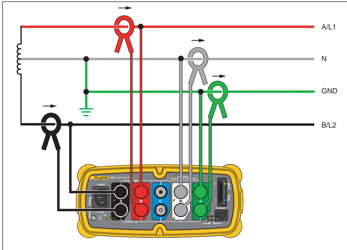
Figura 6. Monofásico-fase dividida
