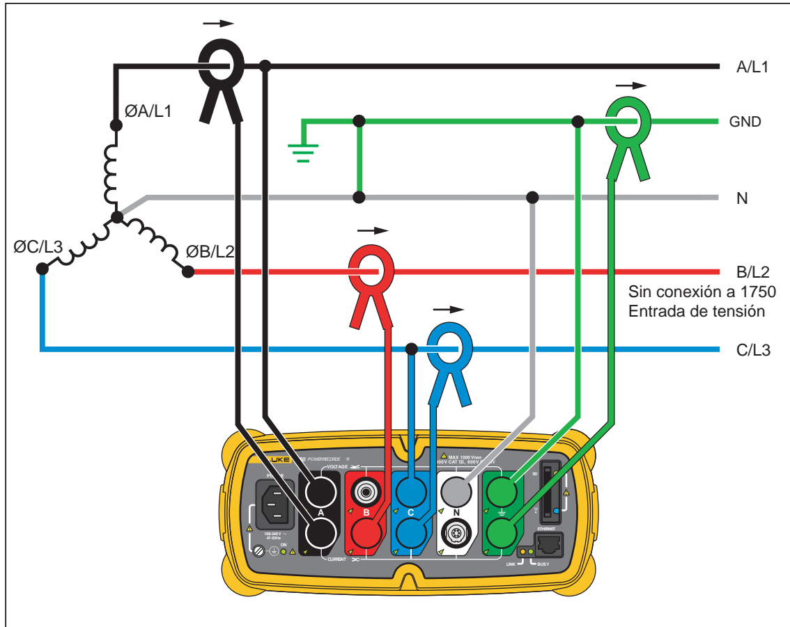
Figura 13. Estrella de 2 ½ elementos
