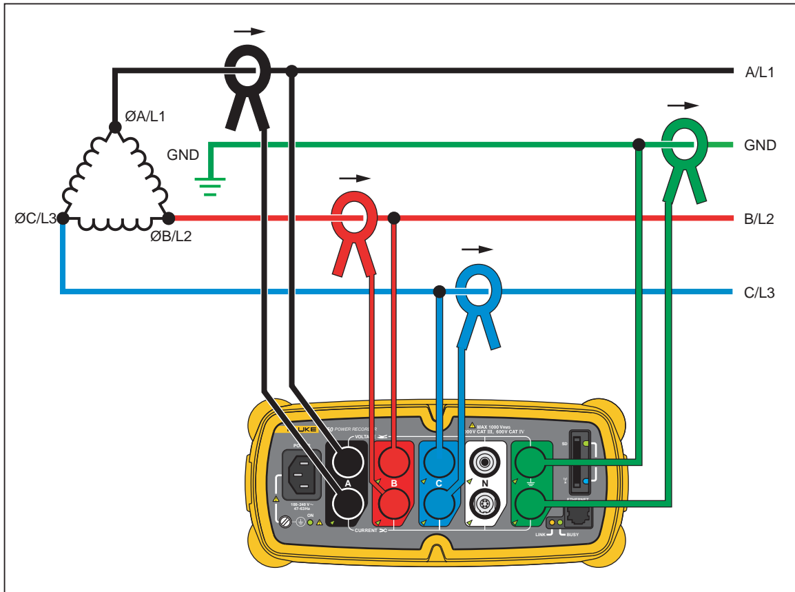
Figura 8. Triángulo trifásico
