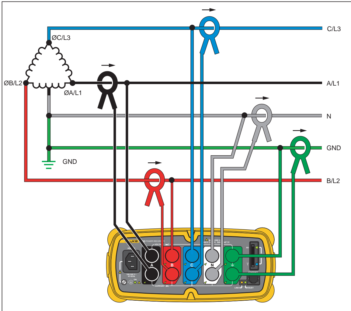
Figura 10. Patilla larga trifásico
