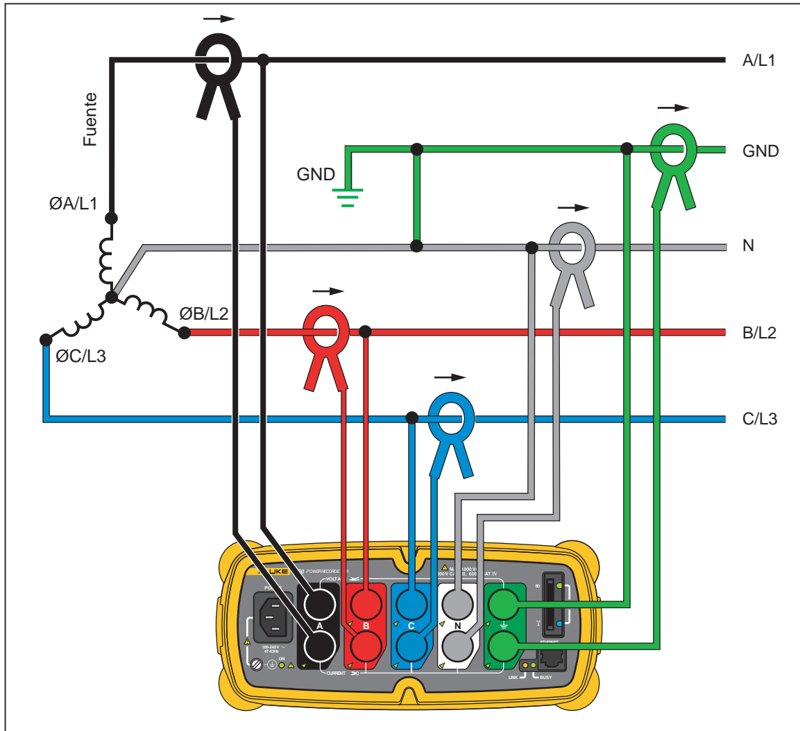
Figura 7. Estrella trifásico
