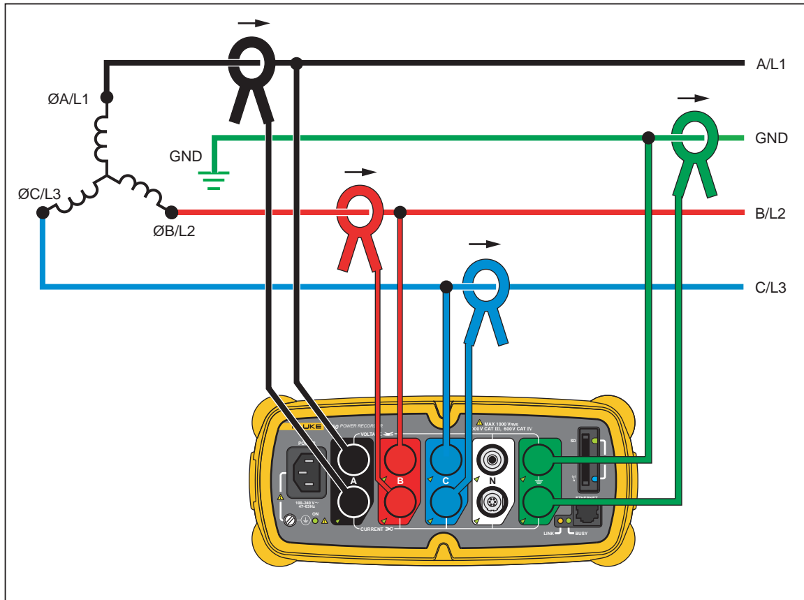
Figura 9. TI trifásico
