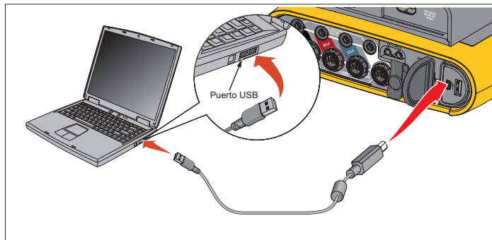
Figura 13. Conexiones del Power Logger con el PC
