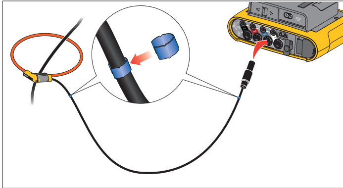
Figura 5. Cables de prueba con código de color
