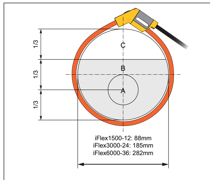
Figura 14. Ventana de la sonda iFlex
