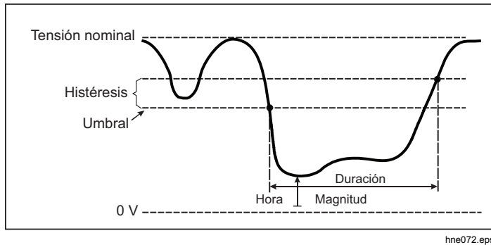
Figura 10. Características de una interrupción de tensión
