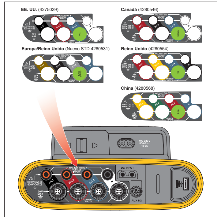
Figura 7. Etiqueta de panel de conectores
