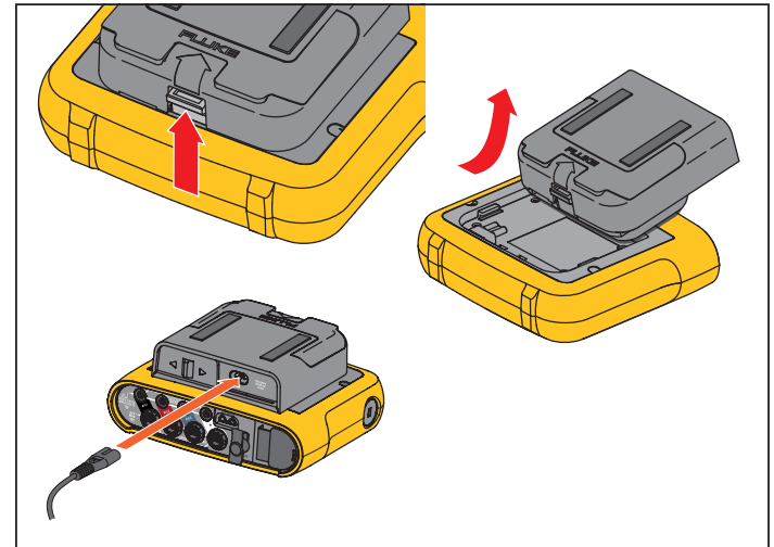
Figura 6. Fuente de alimentación y batería
