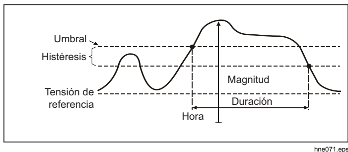
Figura 8. Características de una sobretensión
