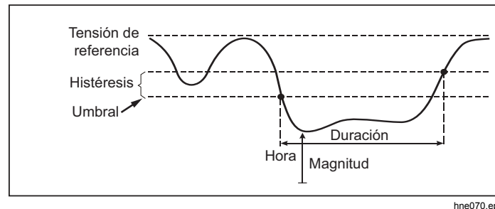
Figura 9. Características de una caída de tensión
