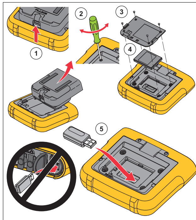
Figura 2. Instalación del adaptador
