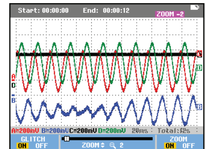
Capture detalles de forma de onda de alta resolución durante periodos prolongados con el modo ScopeRecord™
