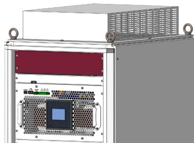
Figura 6: Techo de un SVGm tipo Armario.
