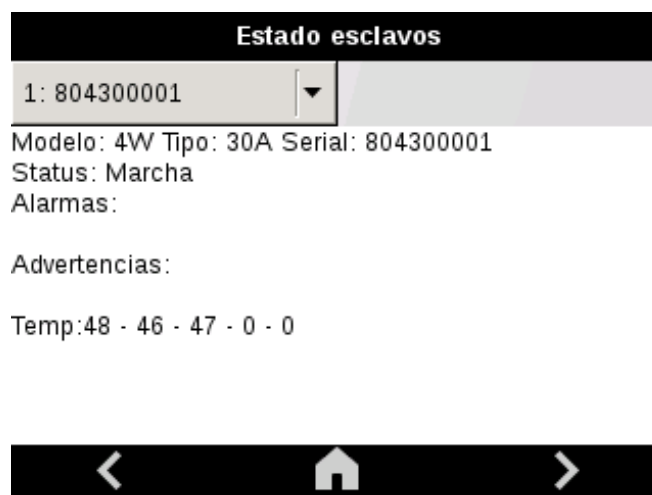
Figura 52: Pantalla de estado de los equipos esclavos (2).
