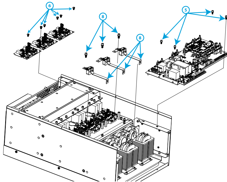
Figura 78:SVGm-xxx-100R cambio ventiladores (Paso 5, 6, 8).
