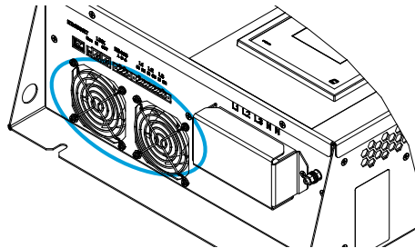
Figura 70: Situación de los ventiladores de refrigeración.
