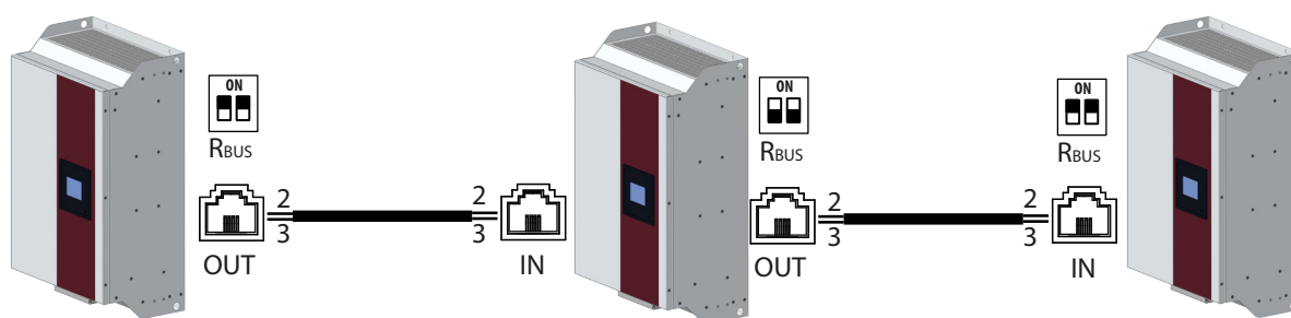
Figura 28: Conexión de 3 equipos en paralelo, mediante el cable de comunicaciones.
