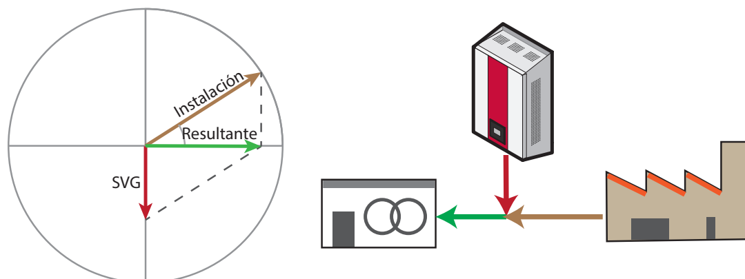
Figura 31: Funcionamiento del SVGm.
