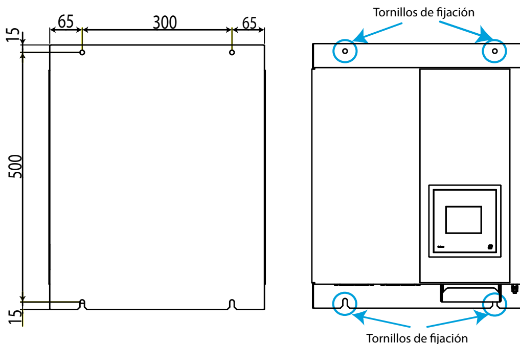
Figura 5: Instalación SVGm tipo Mural.
