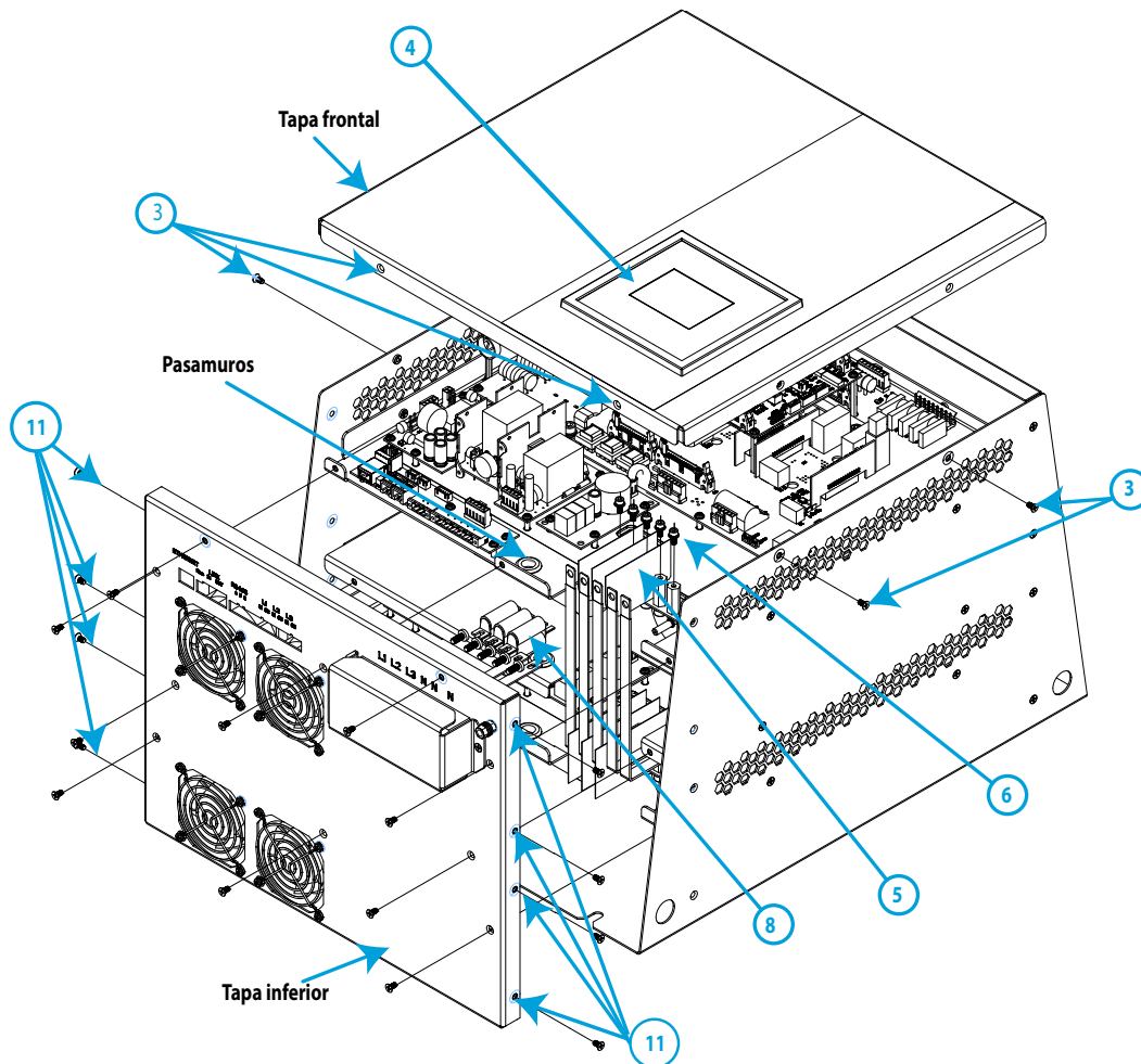
Figura 74: Pasos para realizar el cambio de ventiladores (parte 1).
