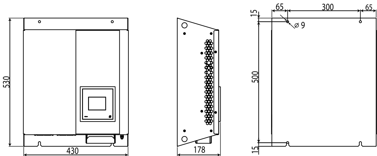
Figura 83: Dimensiones SVGm-xxx-030M.
