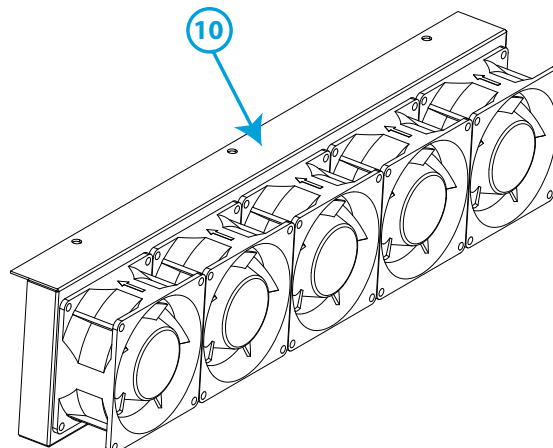
Figura 80:SVGm-xxx-100R cambio ventiladores (Paso 10).
