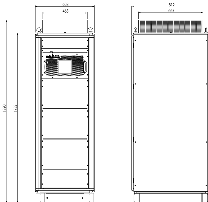
Figura 87: Dimensiones SVGm tipo armario.
