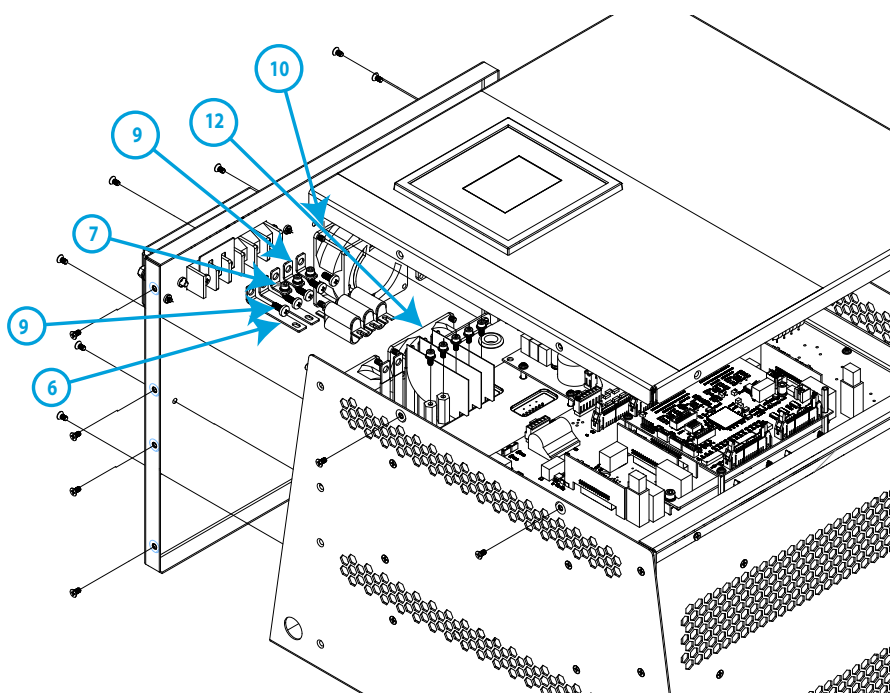
Figura 75: Pasos para realizar el cambio de ventiladores (parte 2).
