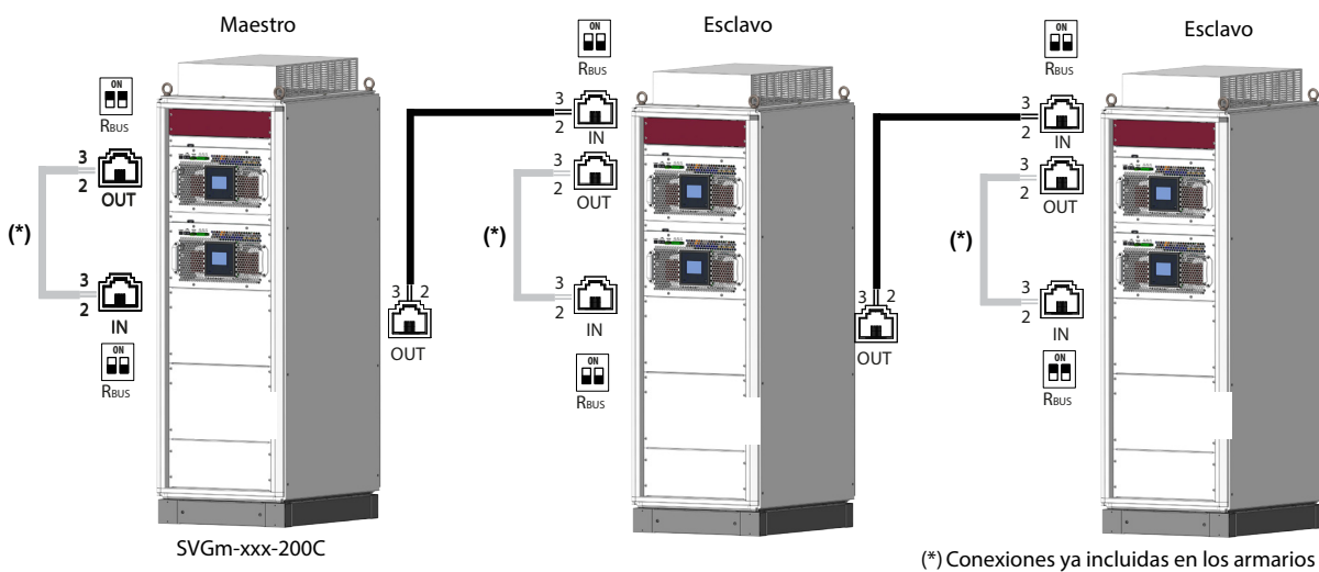
Figura 29: Conexión de 3 equipos en paralelo, mediante el cable de comunicaciones (Maestro SVGm 200 kvar).
