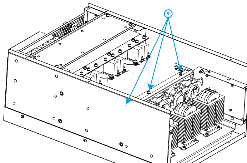
Figura 79:SVGm-xxx-100R cambio ventiladores (Paso 9).
