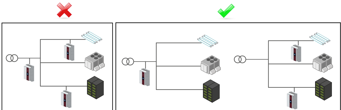
Figura 7: No instalar varios generadores estáticos en serie.
