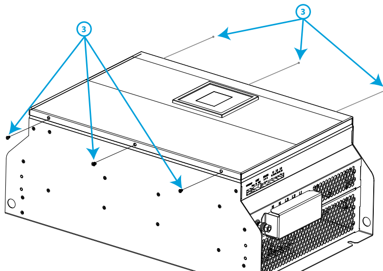
Figura 81:SVGm-xxx-100M cambio ventiladores (Paso 3).
