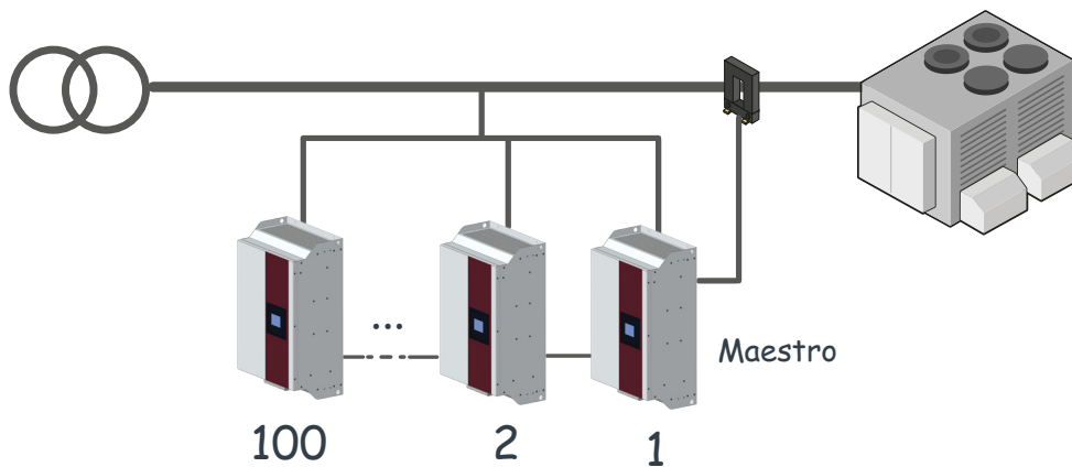
Figura 27: Conexión de 2 a 100 generadores estáticos en paralelo (Transformadores en lado carga).
