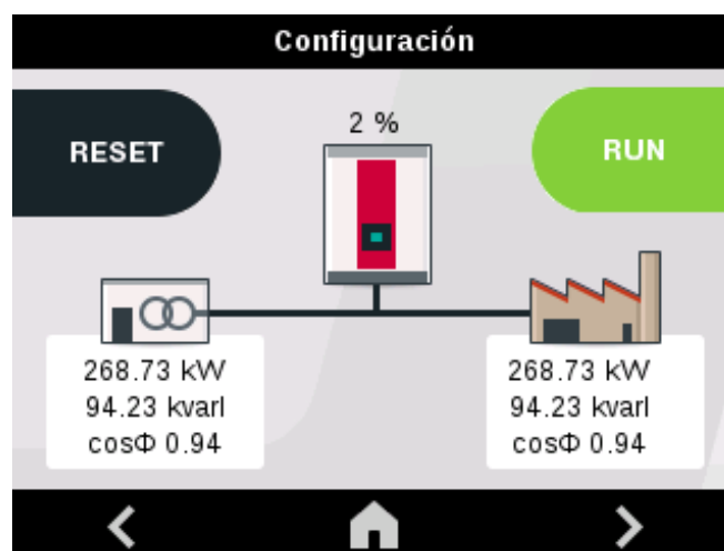
Figura 32: Display.
