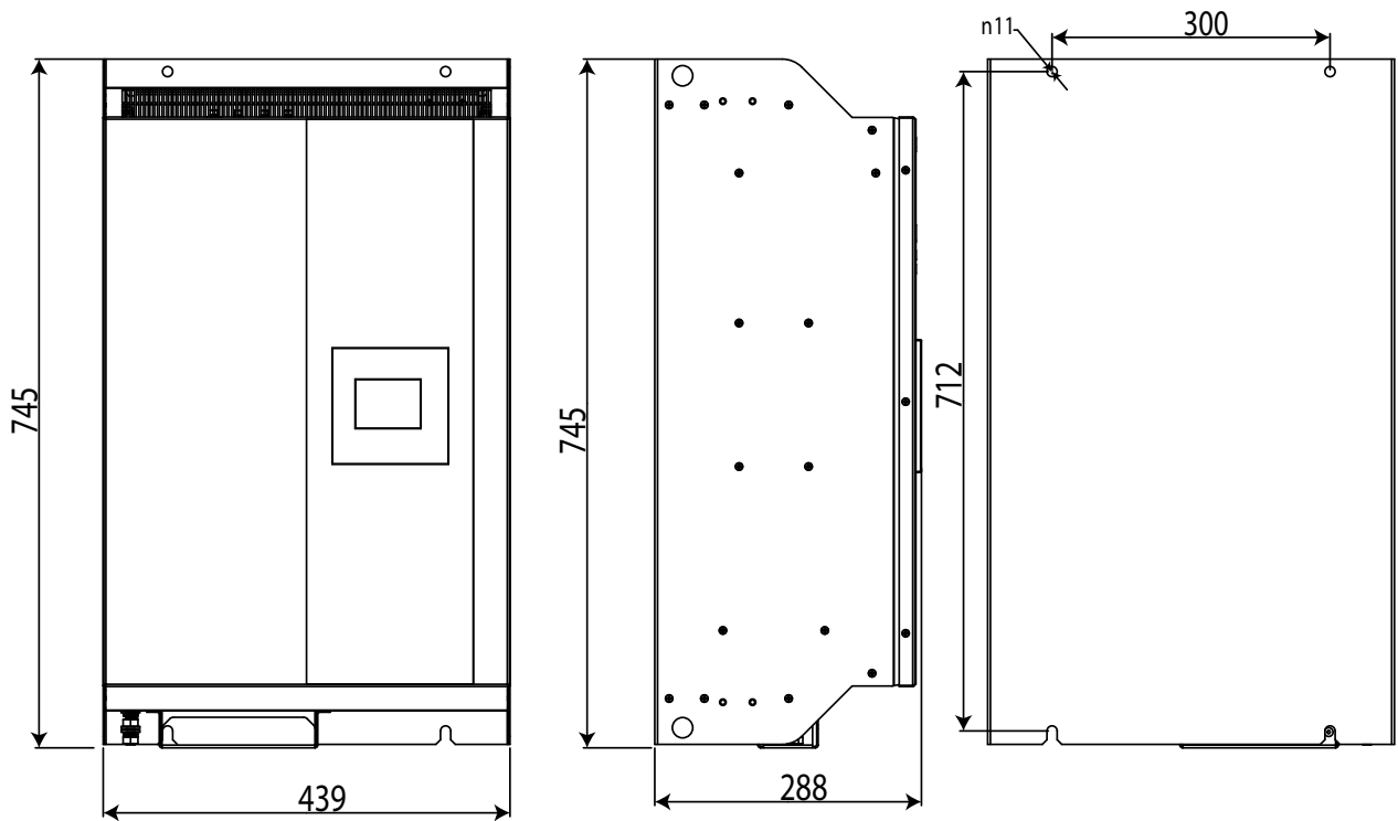
Figura 85: Dimensiones SVGm-xxx-100M
