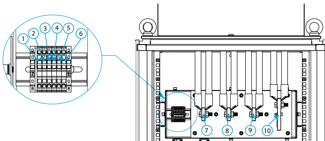
Figura 18: Bornes SVGm tipo Armario (Conexiones en la parte superior).
