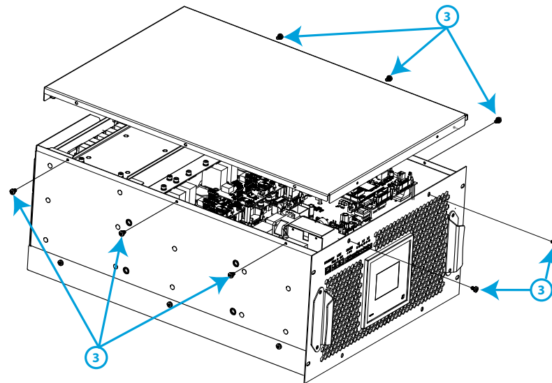
Figura 76:SVGm-xxx-100R cambio ventiladores (Paso 3).
