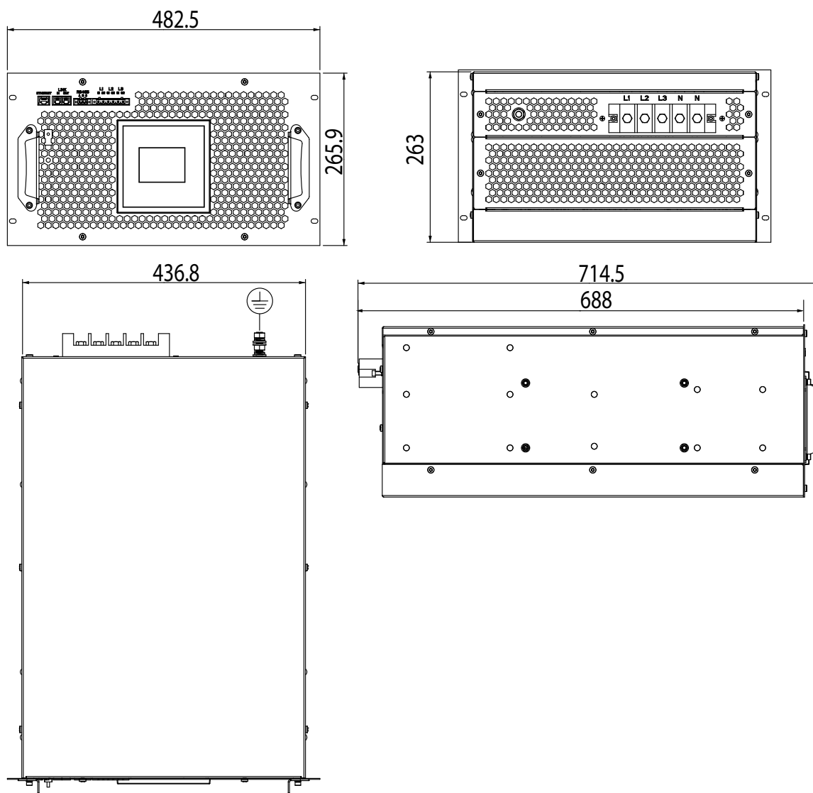
Figura 86: Dimensiones SVGm-xxx-100R.
