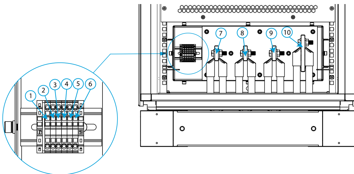
Figura 17: Bornes SVGm tipo Armario (Conexiones en la parte inferior).
