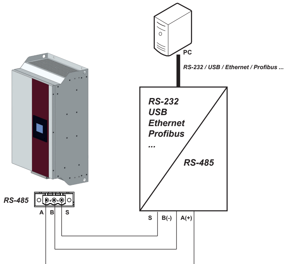
Figura 65: Esquema de conexionado RS-485.
