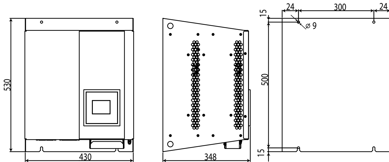
Figura 84: Dimensiones SVGm-xxx-060M
