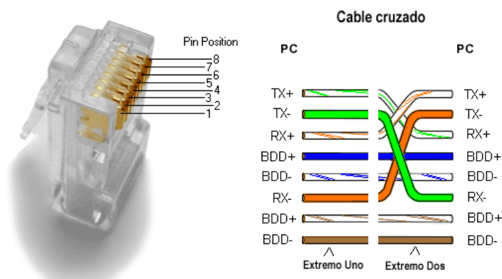
Figura 66: Conector RJ-45 : Diagrama de conexión Ethernet cruzado.
