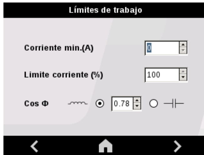
Figura 58: Pantalla de configuración: Límites de trabajo.
