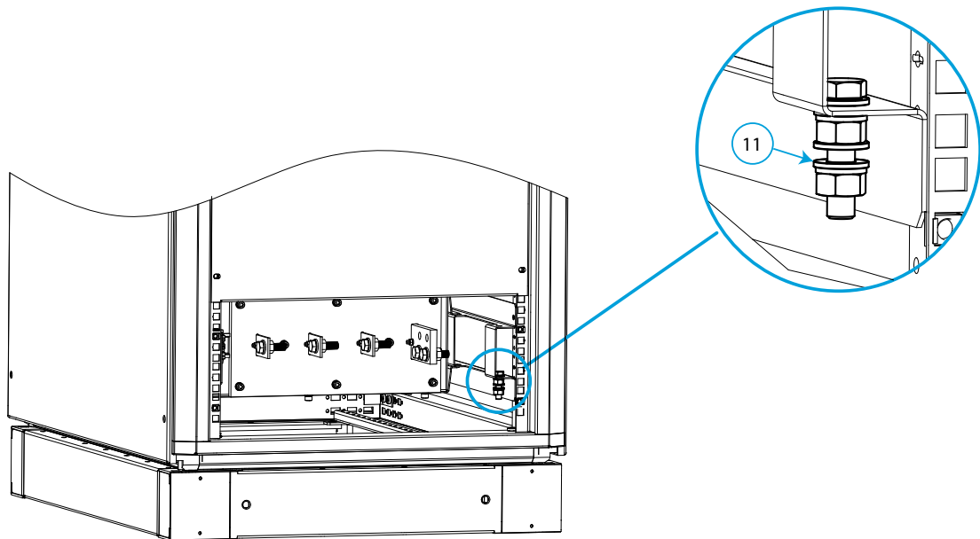
Figura 19: Borne de tierra en SVGm tipo Armario.
