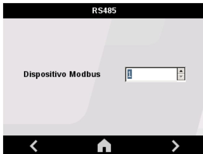
Figura 61: Pantalla de configuración: Comunicaciones RS-485.
