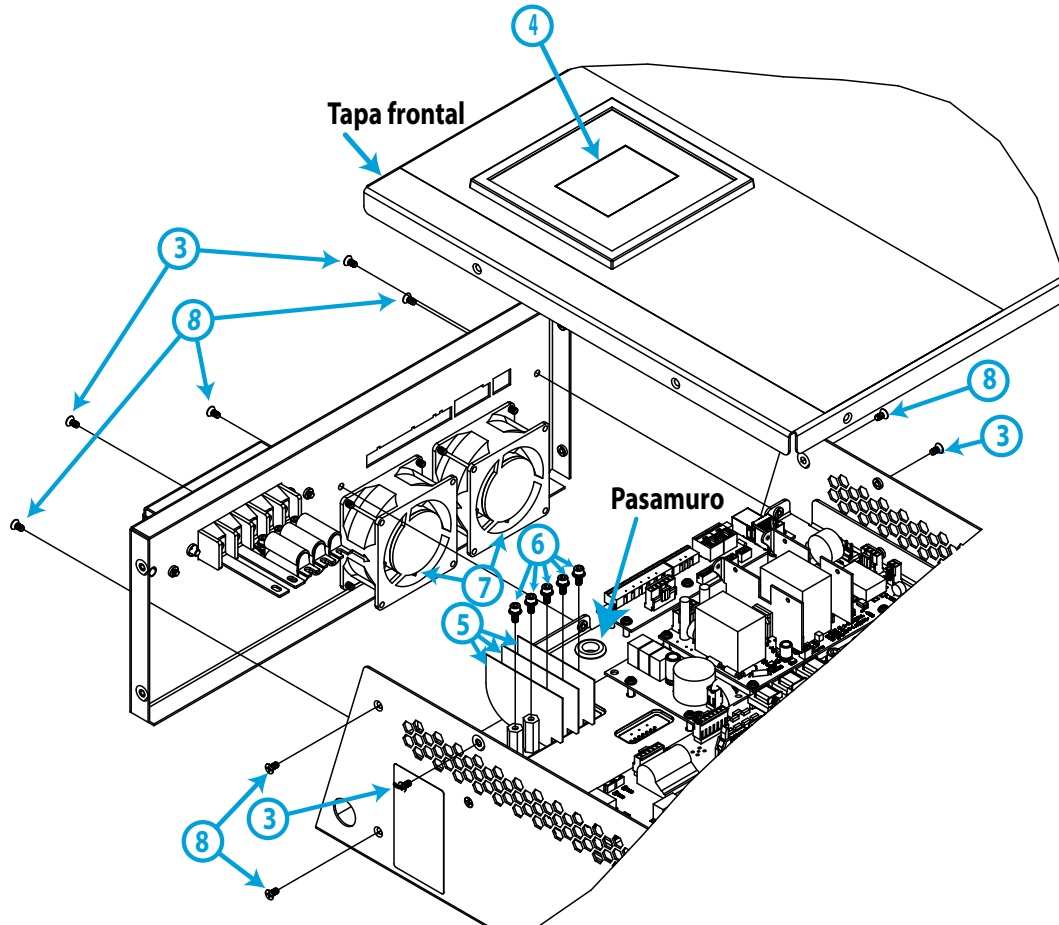
Figura 71:Pasos para realizar el cambio de ventiladores.
