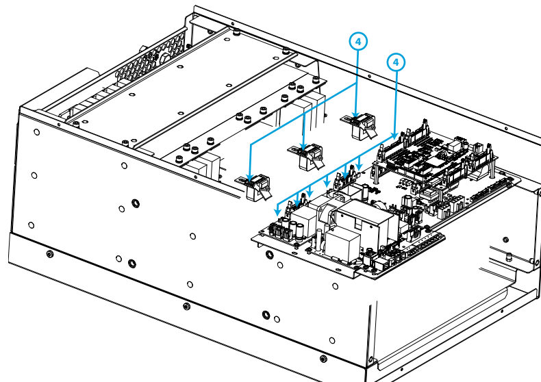
Figura 77:SVGm-xxx-100R cambio ventiladores (Paso 4).
