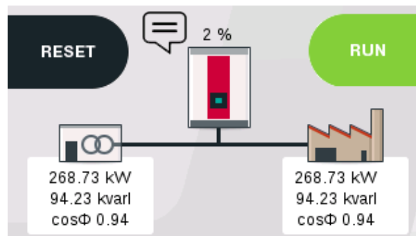
Figura 34: Área central.
