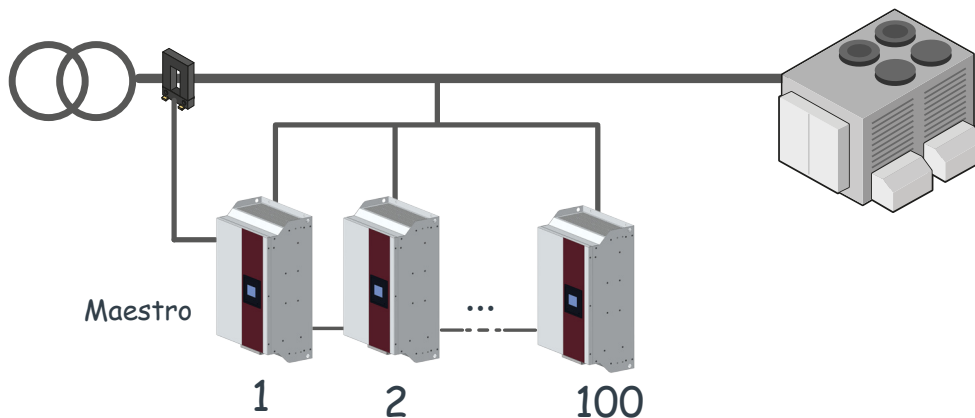
Figura 26: Conexión de 2 a 100 generadores estáticos en paralelo (Transformadores en lado red).
