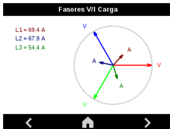
Figura 43: Fasores de Carga.
