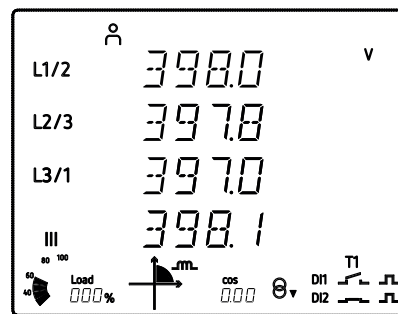
Figura 22: Pantalla del CVM-C11 con el perfil de funcionamiento usuario.
