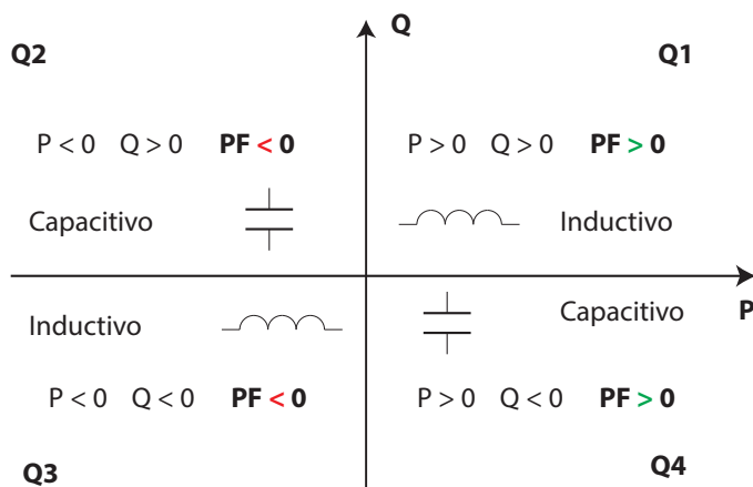
Figura 10: Convenio de medida IEC 61557-12.
