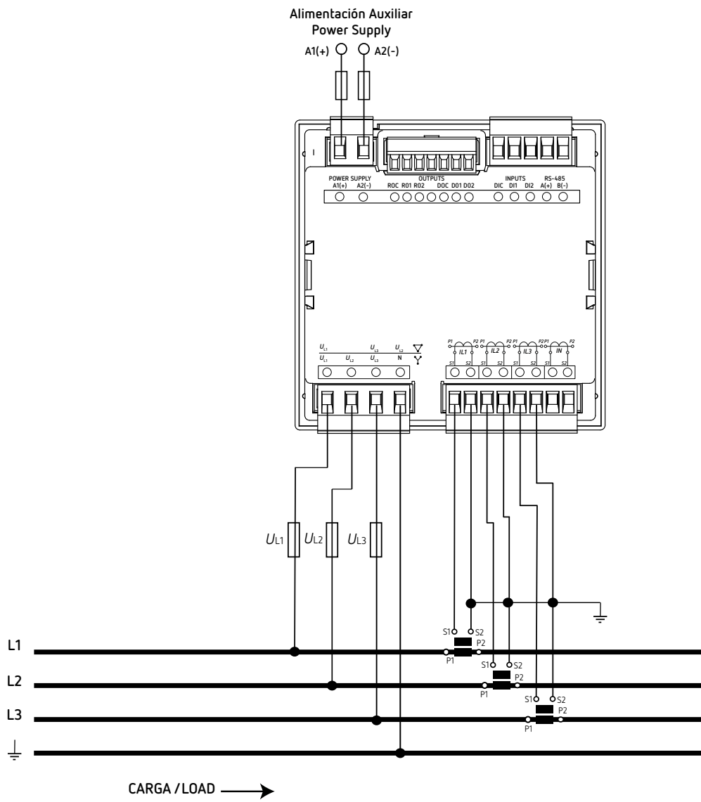
Figura 8: Medida trifásica con conexión a 3 hilos y tierra.
