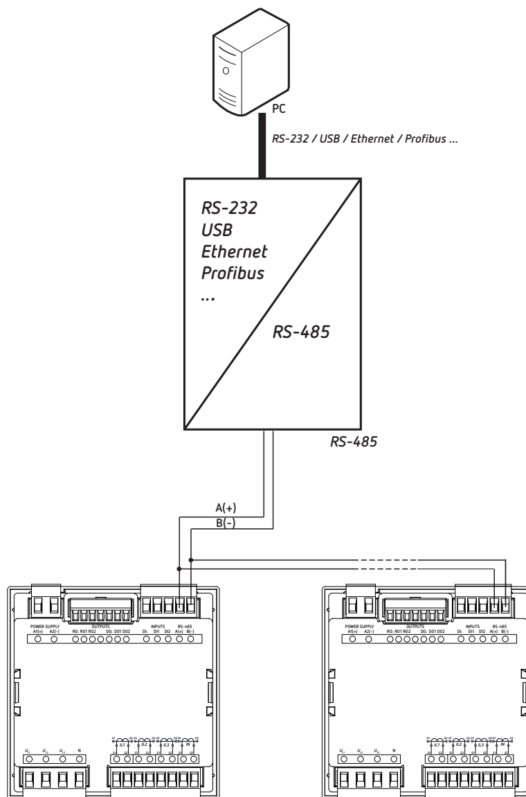
Figura 24: Esquema de conexionado RS-485.
