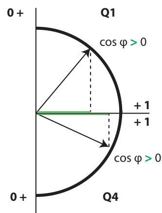
Figura 10: Convenio de medida IEC 61557-12.
