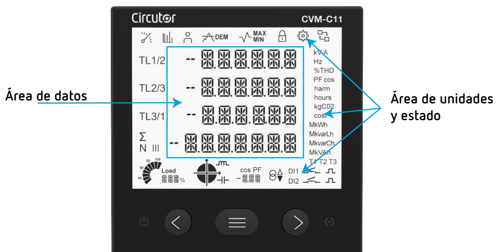
Figura 14: Áreas del display del CVM-C11.
