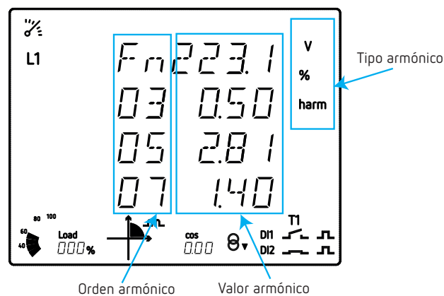
Figura 23: Pantalla de los armónicos del CVM-C11.
