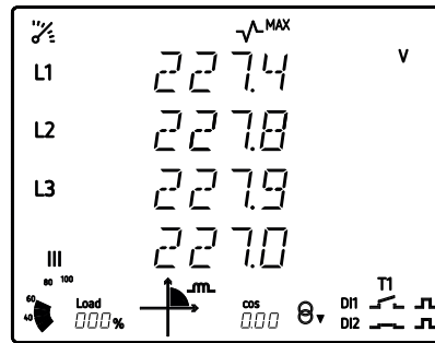
Figura 20: Pantalla del perfil analizador visualizando los valores máximos.
