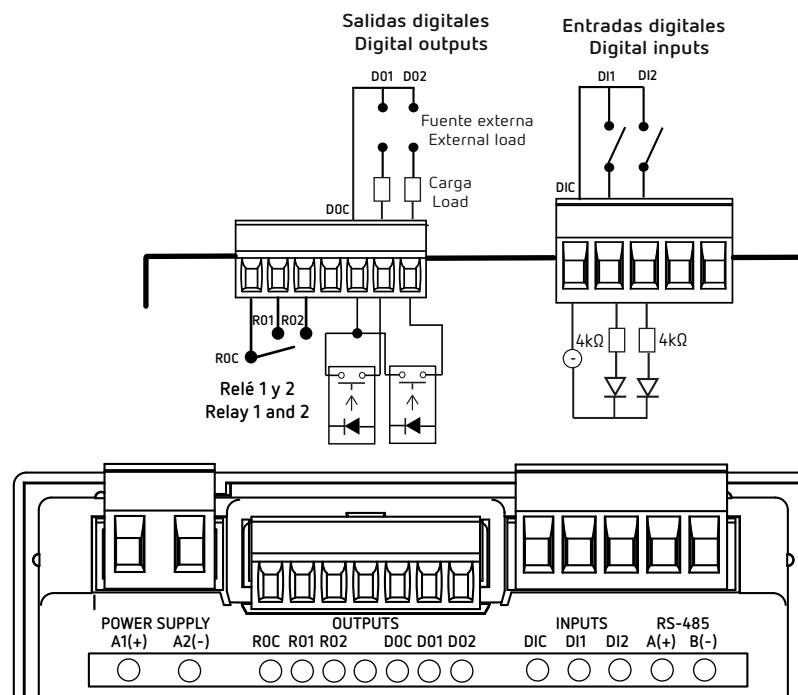
Figura 19: Relés, Salidas digitales y Entradas digitales.
