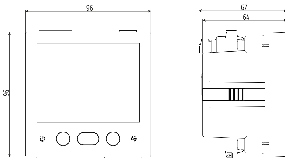
Figura 25: Dimensiones del CVM-C11.
