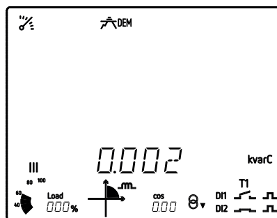
Figura 21: Pantalla del perfil analizador visualizando los valores de máxima demanda.
