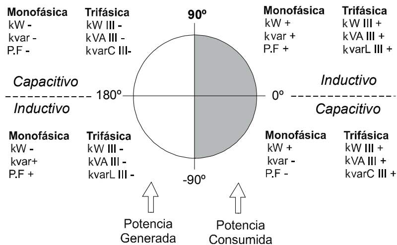
Figura 9: Convenio de medida CIRCUITOR.
