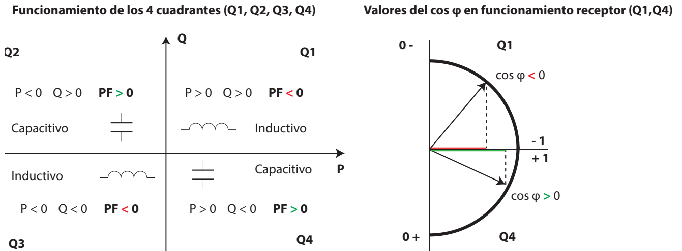
Figura 11: Convenio de medida IEEE 1459.
