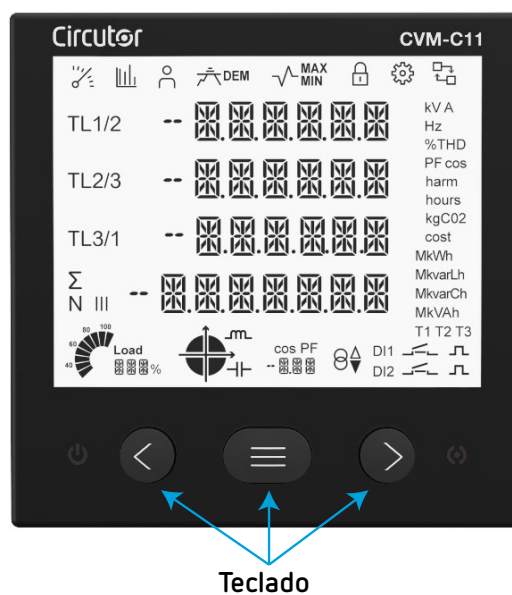
Figura 17: Teclado del CVM-C11.
