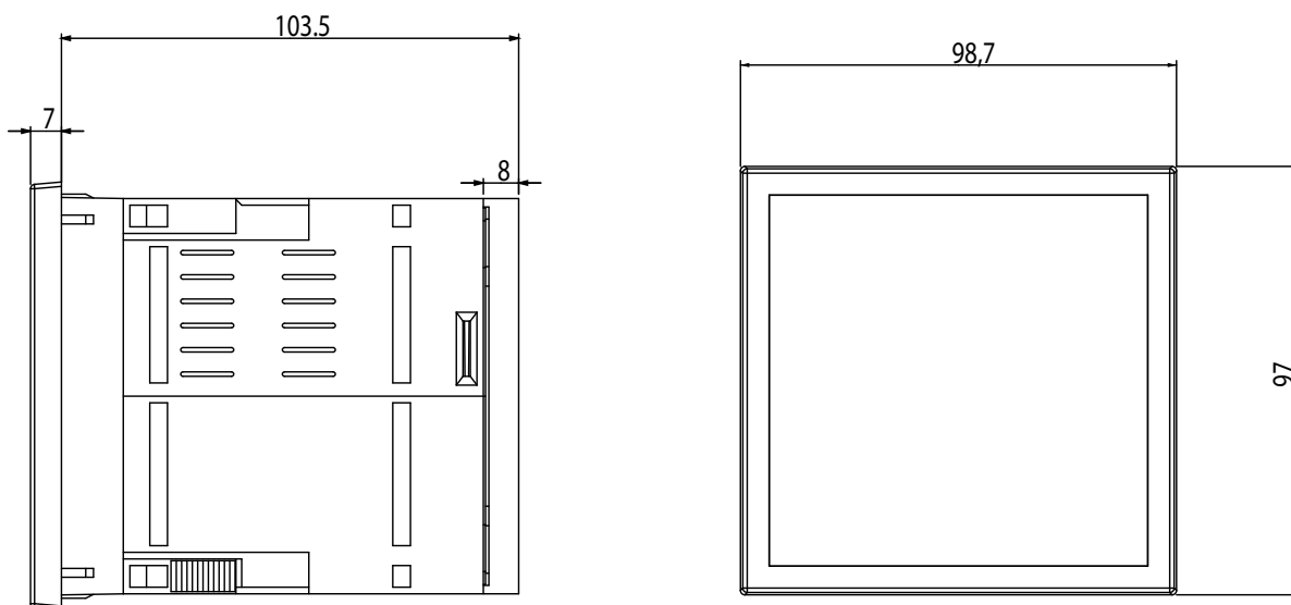
Figura 140: Dimensiones CVM-B100.
