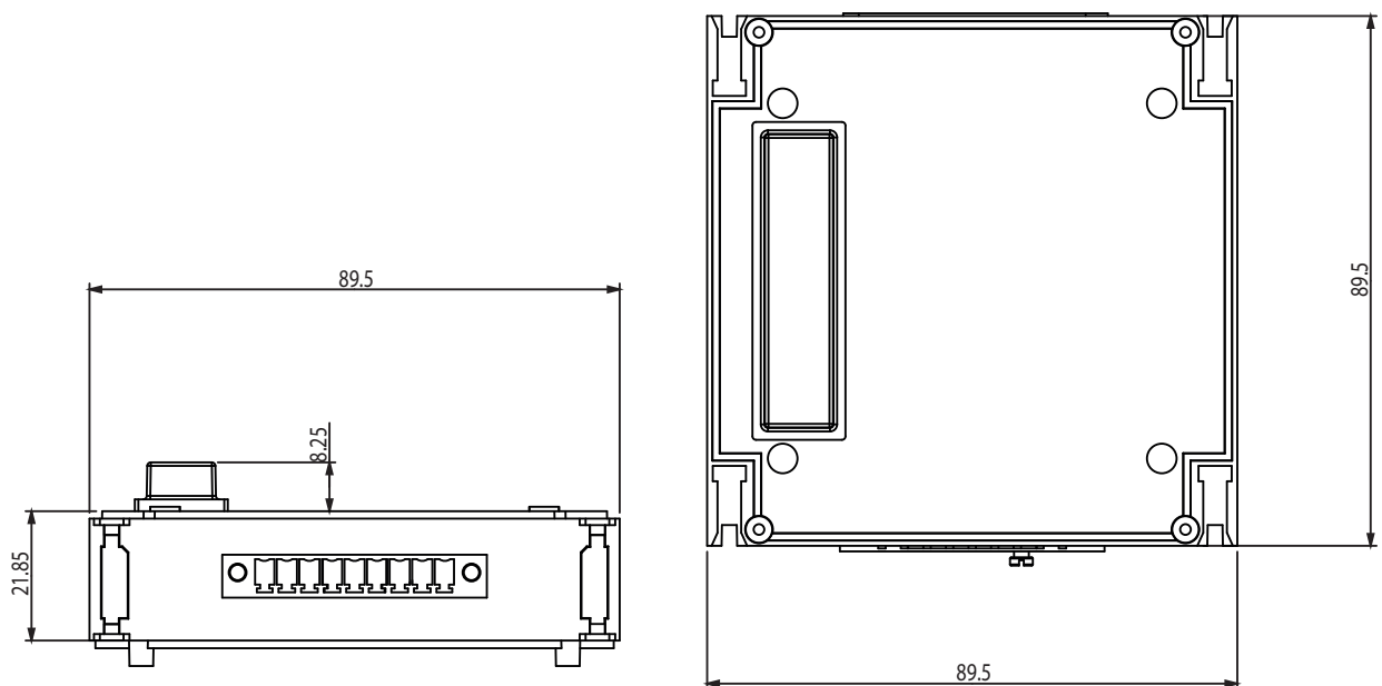
Figura 142: Dimensiones módulo de expansión.
