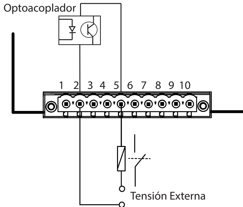
Figura 120: Esquema de conexionado, salida digitales de transistor.
