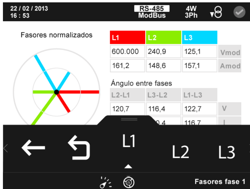
Figura 63: Pantalla de visualización de fasores normalizados.
