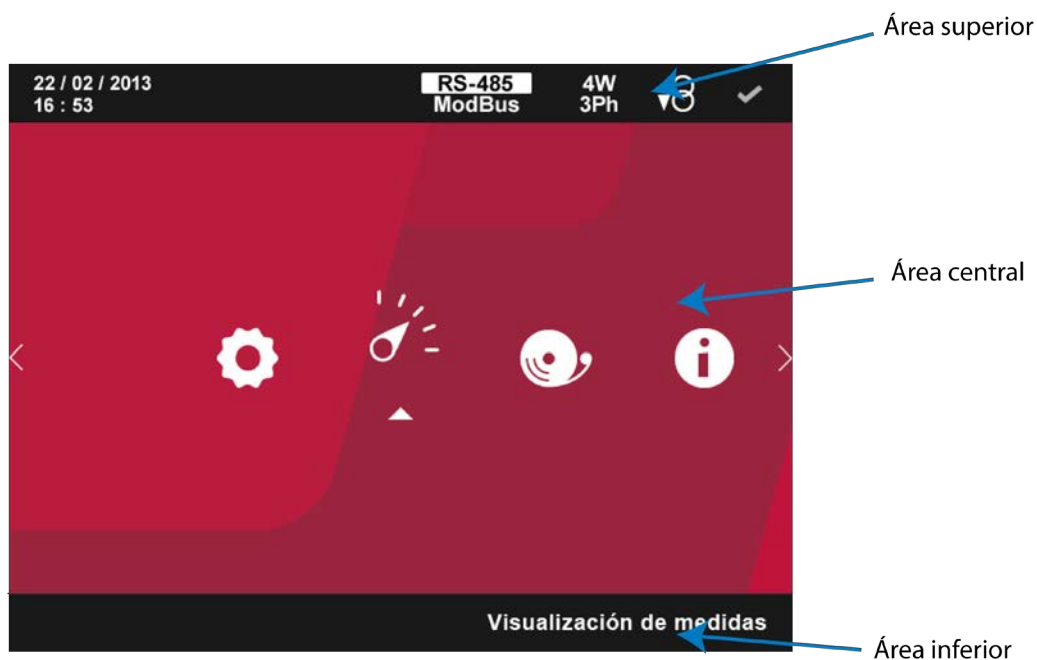
Figura 19: Áreas del display del CVM-B.
