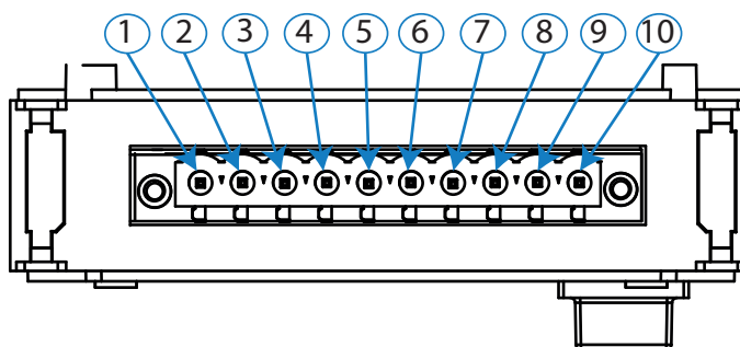
Figura 116: Bornes Entradas/Salidas digitales de Relé, cara superior.
