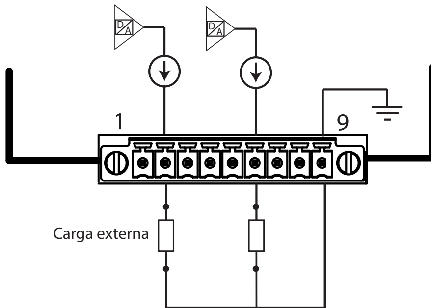
Figura 124: Esquema de conexionado, salidas analógicas.
