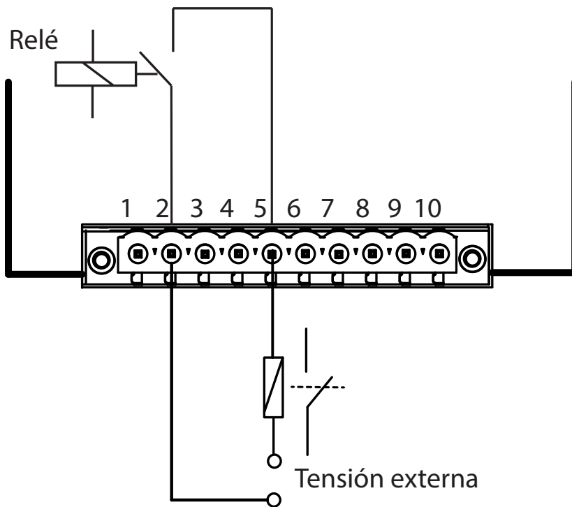
Figura 122: Esquema de conexionado, salida digitales de transistor.
