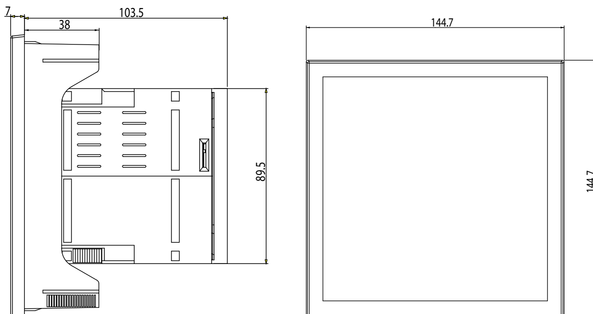
Figura 141: Dimensiones CVM-B150.
