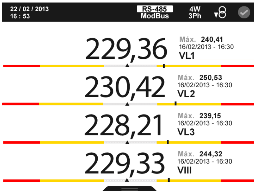
Figura 54: Parámetros instantáneos (visualizar 4 parámetros).
