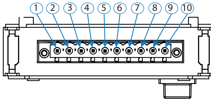
Figura 114: Bornes Entradas/Salidas digitales de Transistor, cara superior.
