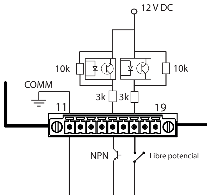
Figura 121: Esquema de conexionado, entradas digitales.
