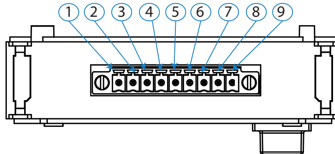
Figura 118: Bornes Entradas/Salidas analógicas, cara superior.
