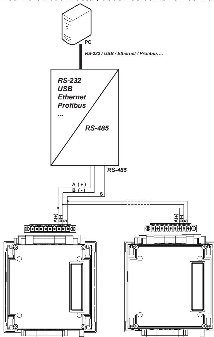
Figura 110: Esquema de conexionado RS-485.
