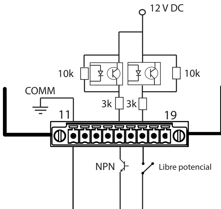
Figura 123: Esquema de conexionado, entradas digitales.
