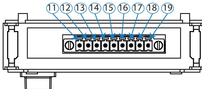
Figura 115:Bornes Entradas/Salidas digitales de Transistor, cara inferior.
