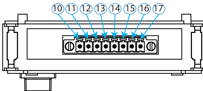
Figura 119: Bornes Entradas/Salidas analógicas, cara inferior.
