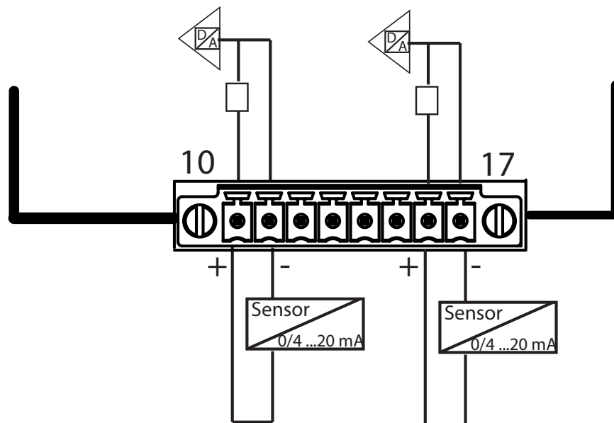
Figura 125: Esquema de conexionado, entradas analógicas.
