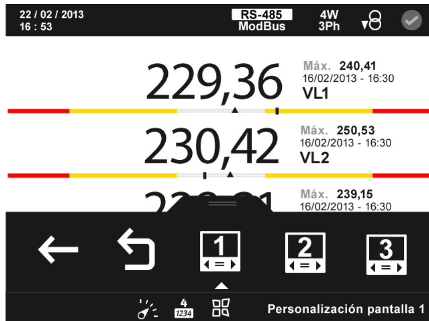
Figura 61: Pantalla de parámetros personalizados (visualizar 4 parámetro).
