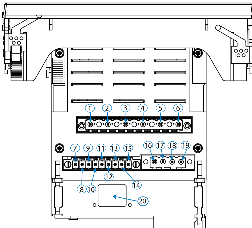
Figura 1:Bornes CVM-A, cara superior.
