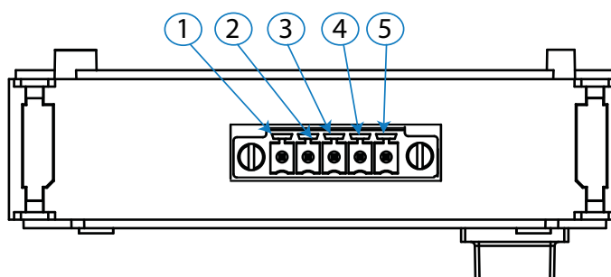
Figura 368: Bornes Módulo de comunicaciones LonWorks.
