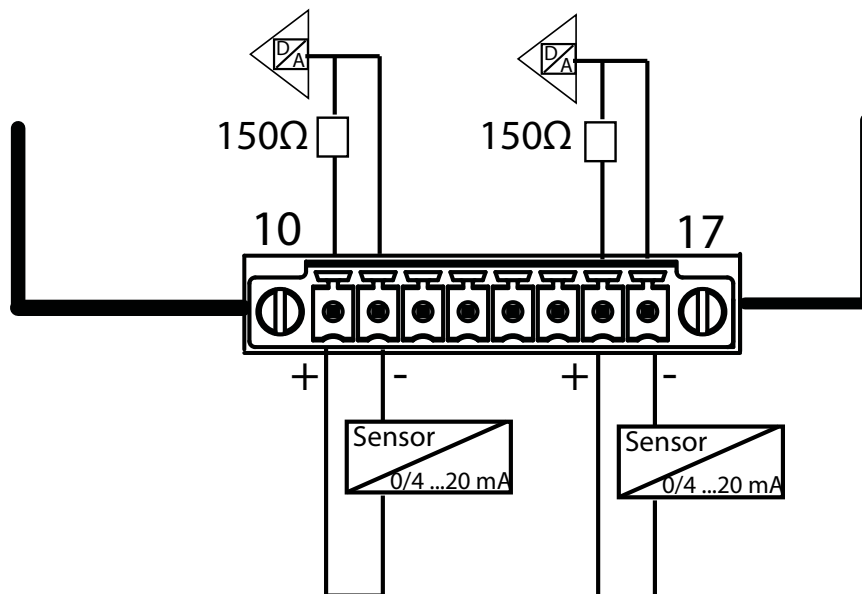
Figura 344: Esquema de conexión, entradas analógicas.
