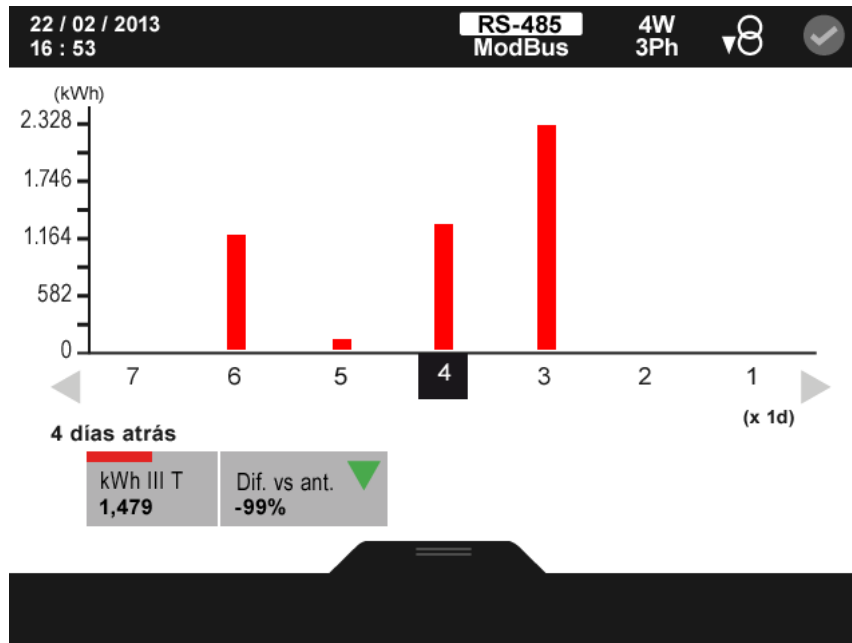
Figura 198:Cierres de la energía activa.
