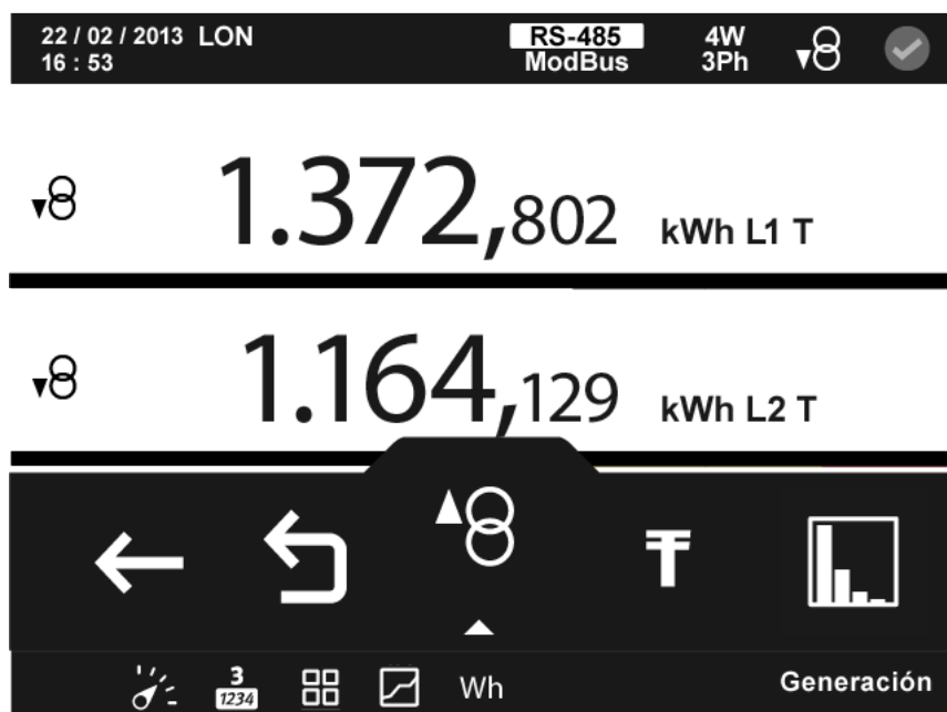
Figura 94: Parámetros incrementales, menú de visualización (visualizar 3 parámetros).
