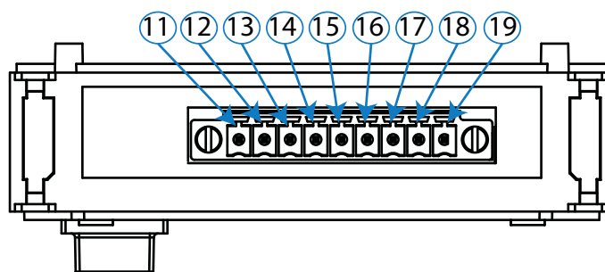
Figura 322: Bornes Entradas/Salidas digitales de Relé, cara inferior.
