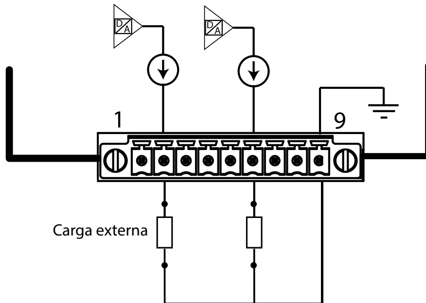
Figura 343: Esquema de conexión, salidas analógicas.
