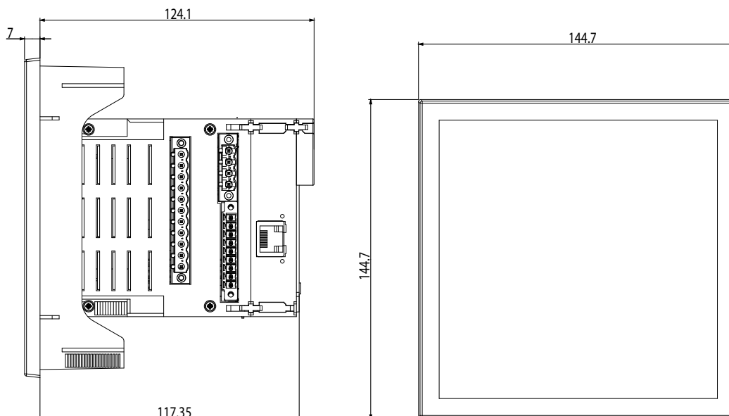
Figura 400: Dimensiones CVM-A1500.
