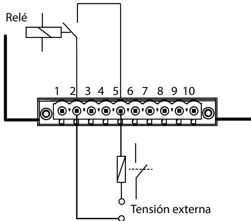
Figura 323: Esquema de conexionado, salida digitales de relé.
