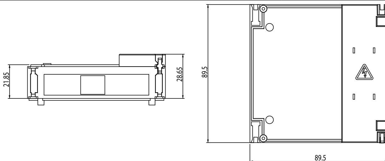
Figura 401: Dimensiones módulo de expansión.
