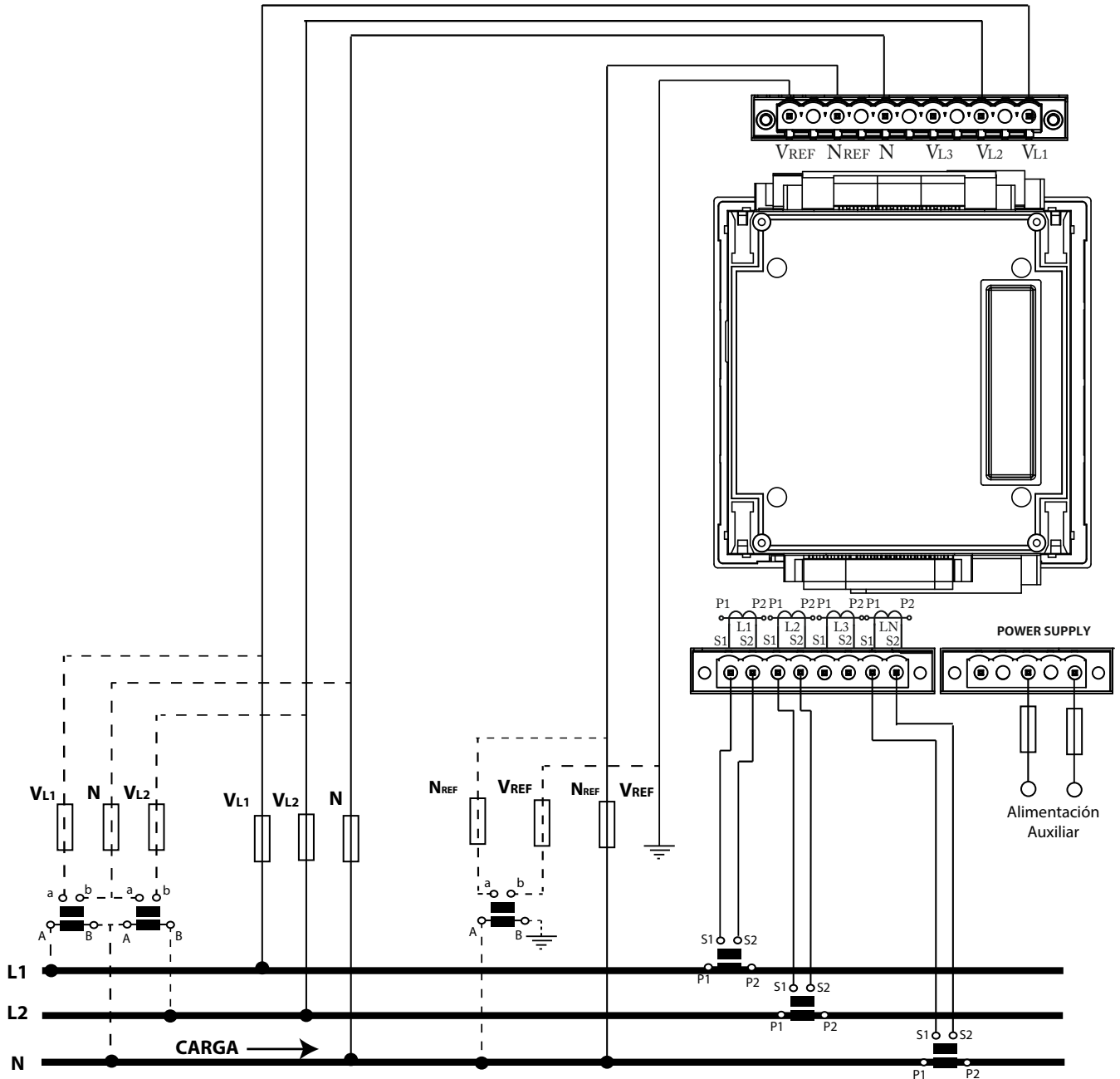
Figura 9: Medida bifásica con conexión a 3 hilos (Secundario del transformador: /1A, /5A o MC1 (/0.250)).
