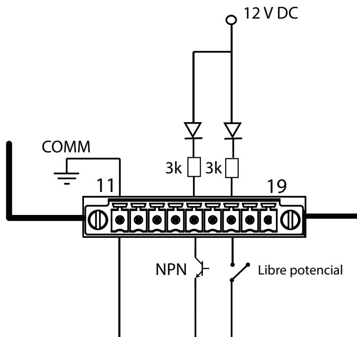
Figura 324: Esquema de conexionado, entradas digitales.
