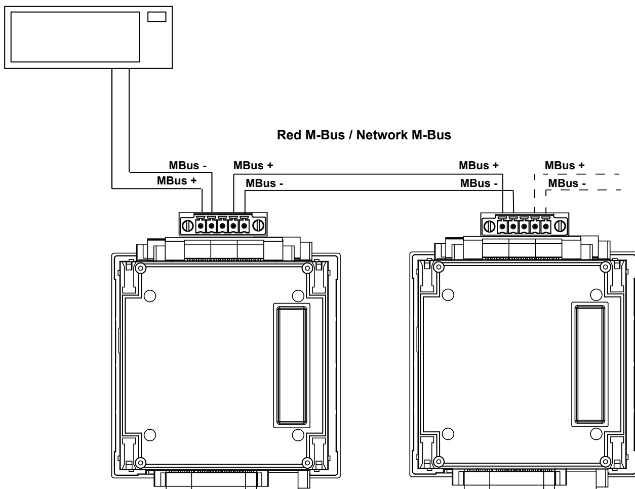
Figura 381: Esquema de conexionado, MBus.
