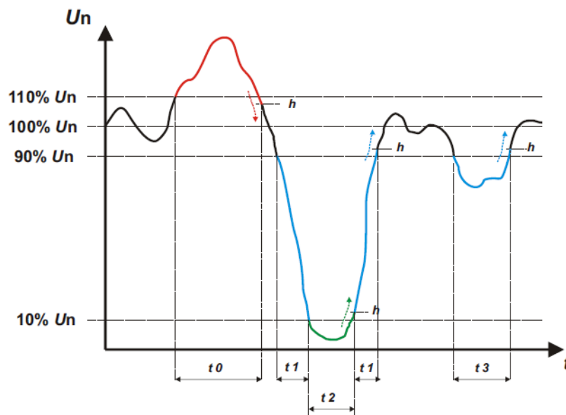
Figura 24: Ejemplo de eventos de Calidad.
