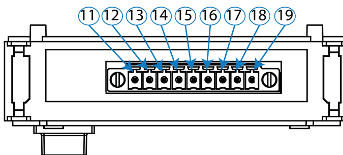
Figura 333:Bornes Entradas/Salidas digitales de Transistor, cara inferior.
