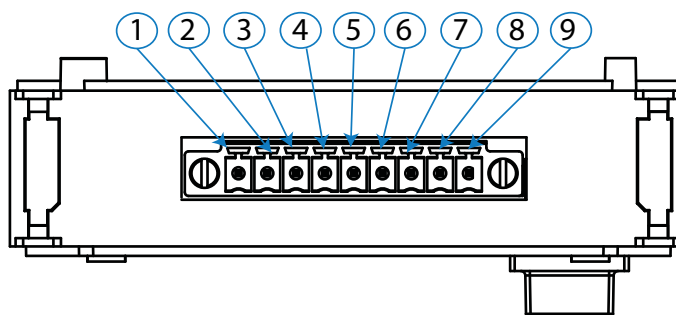
Figura 341: Bornes Entradas/Salidas analógicas, cara superior.
