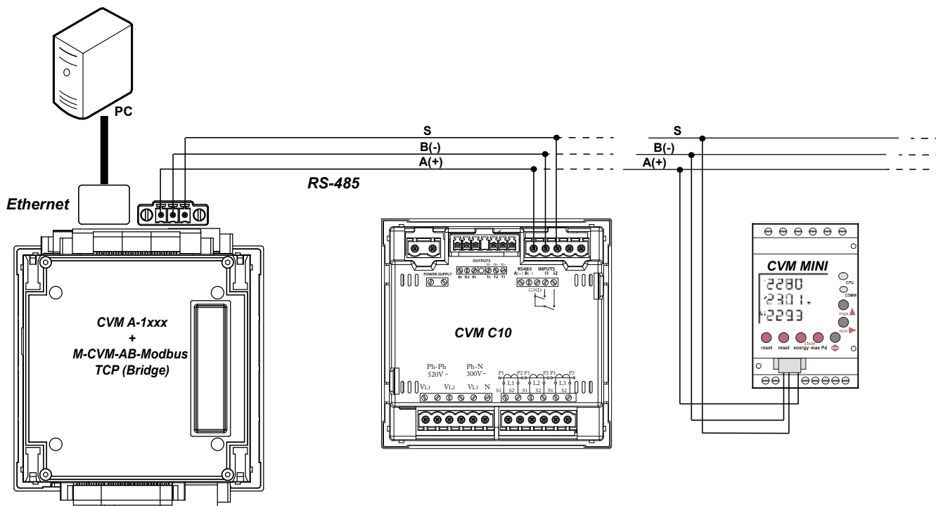
Figura 358:Esquema de conexionado, Modbus TCP (Bridge).
