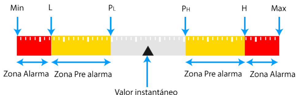
Figura 29: Cálculo de la barra gráfica.
