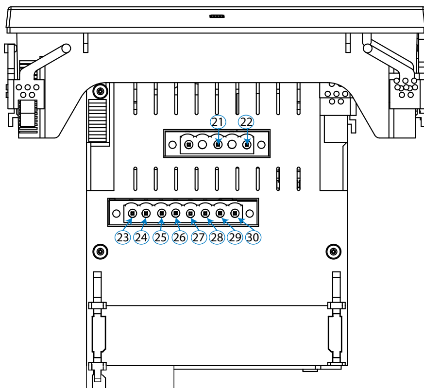
Figura 2: Bornes del CVM-A, cara inferior.
