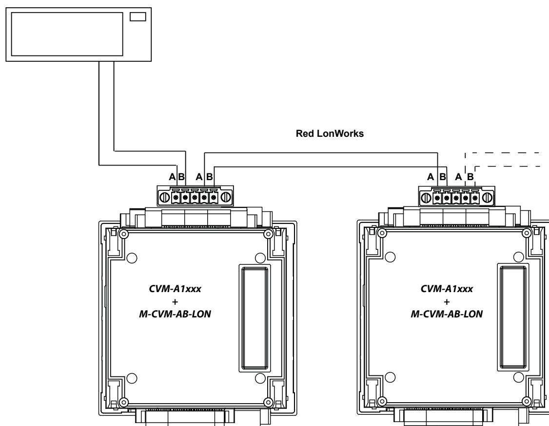
Figura 369: Esquema de conexión, LonWorks.
