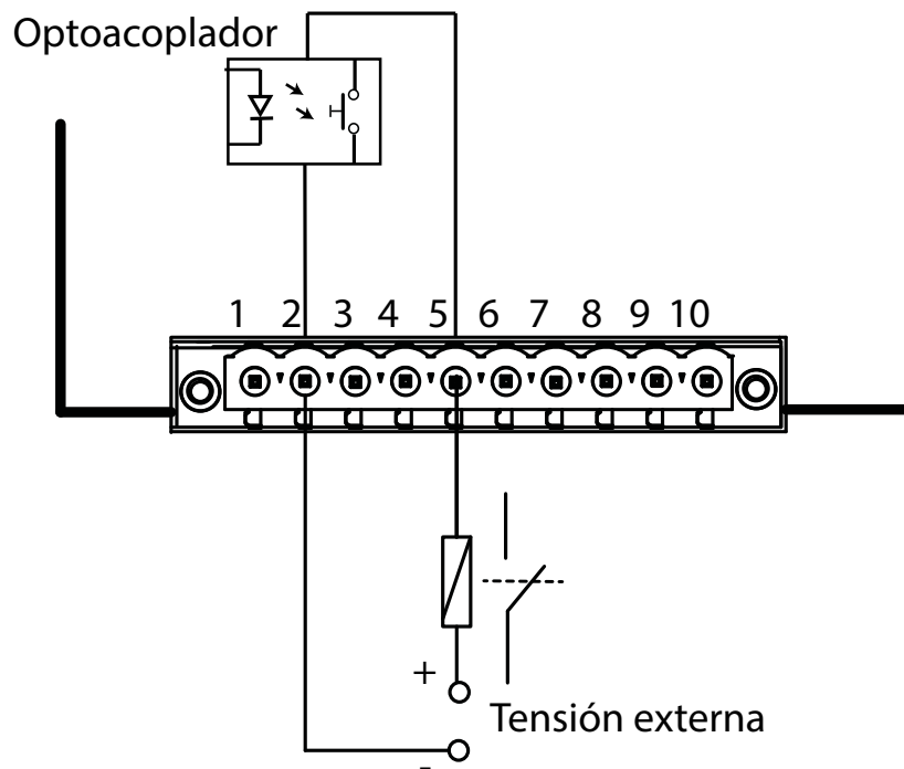
Figura 334: Esquema de conexionado, salida digitales de transistor.
