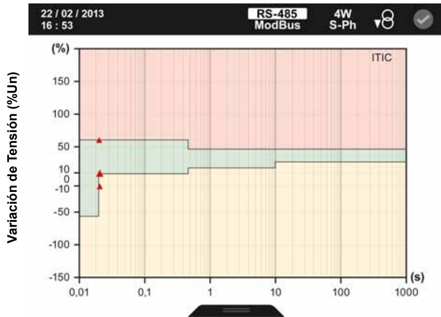
Figura 190: Curva ITIC.
