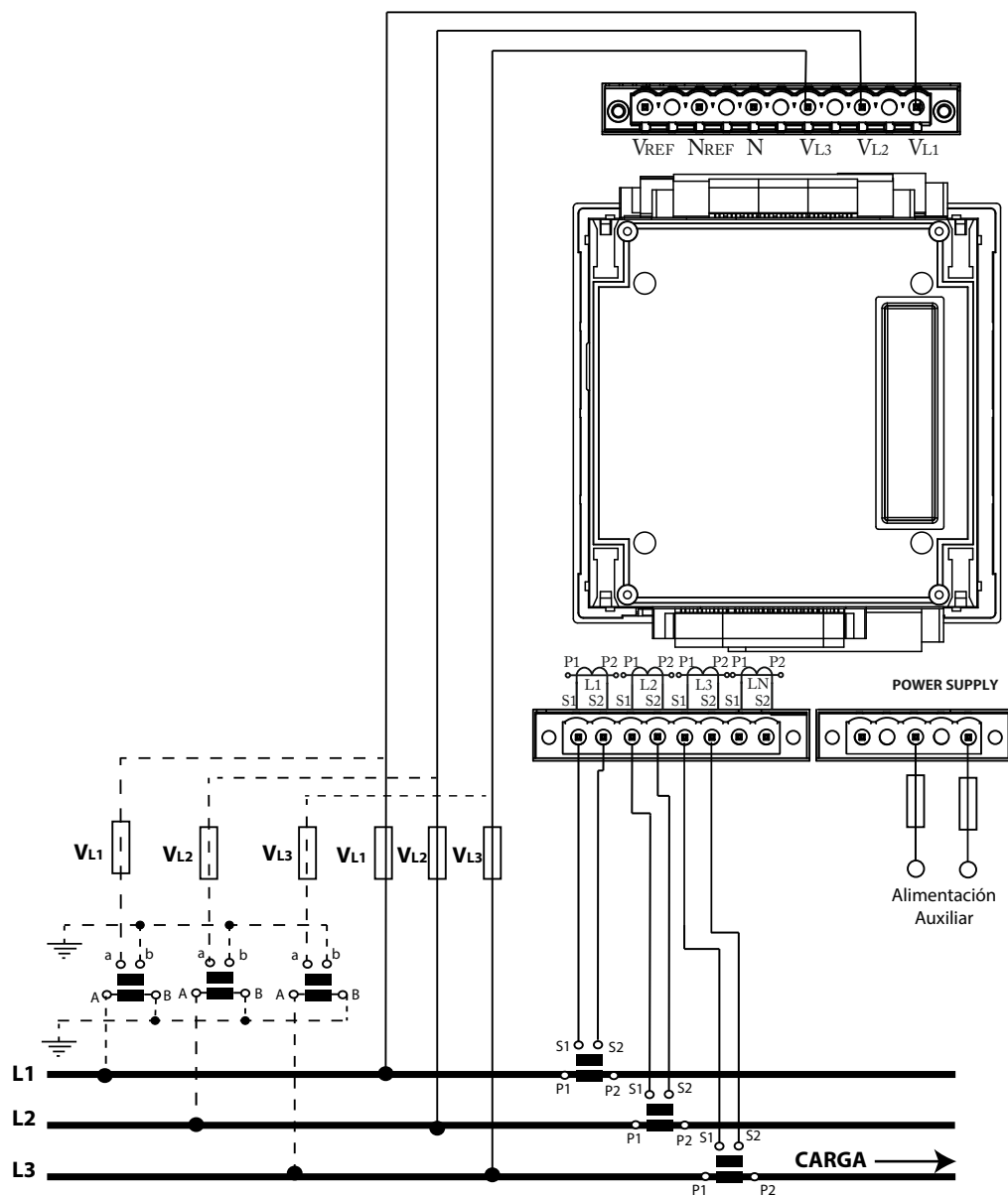
Figura 7: Medida trifásica con conexión a 3 hilos y 3 transformadores de tensión (Secundario del transformador: /1A, /5A o MC1 (/0.250)).
