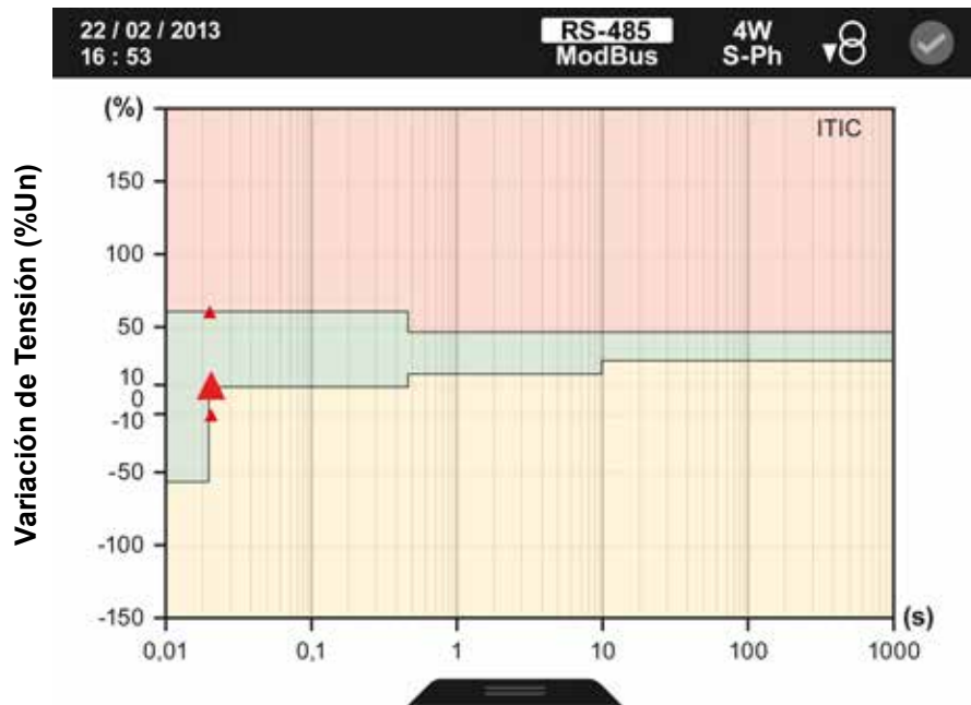
Figura 174: Curva ITIC.
