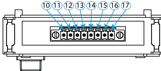
Figura 342: Bornes Entradas/Salidas analógicas, cara inferior.
