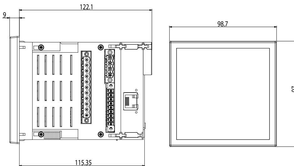
Figura 399: Dimensiones CVM-A1000.
