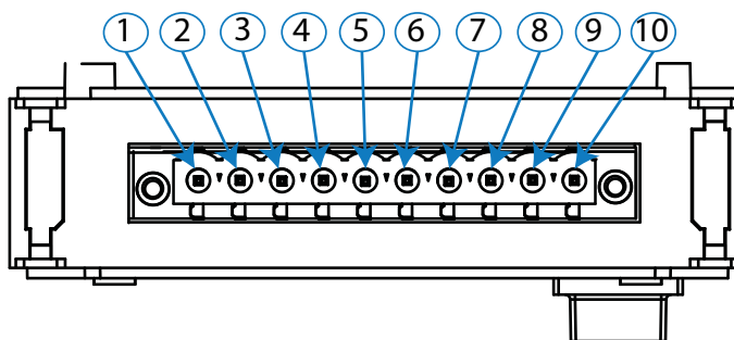
Figura 332: Bornes Entradas/Salidas digitales de Transistor, cara superior.
