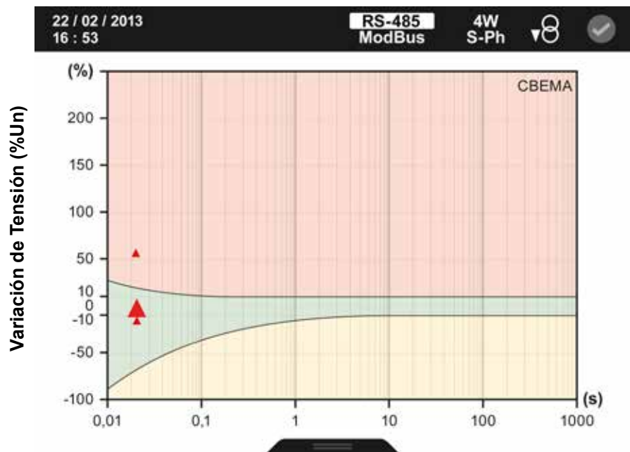
Figura 172: Curva CBEMA.
