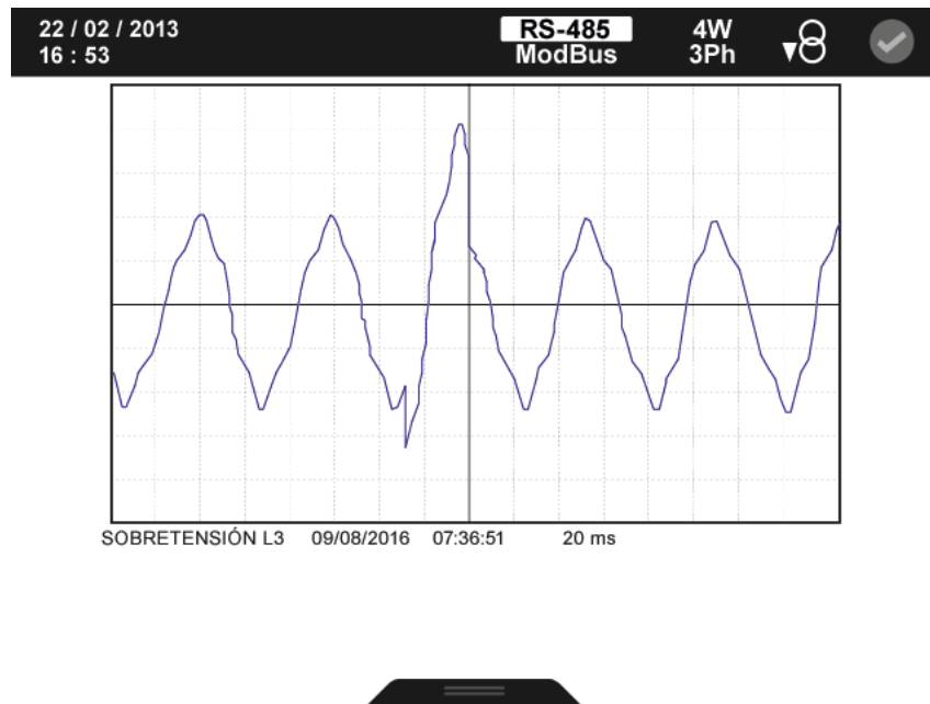
Figura 178: Forma de onda del evento seleccionado.
