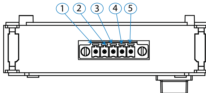
Figura 380: Bornes Módulo de comunicaciones MBus.
