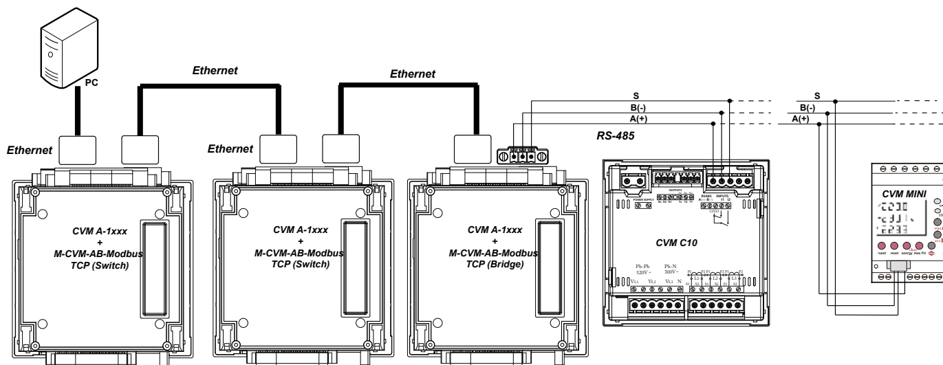
Figura 387:Esquema de conexionado, Modbus TCP (Switch).
