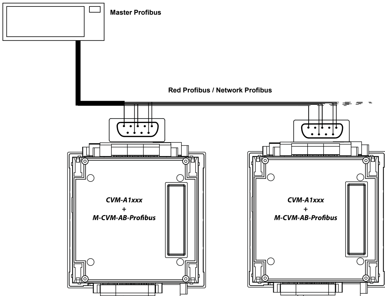
Figura 376:Esquema de conexionado, Profibus.
