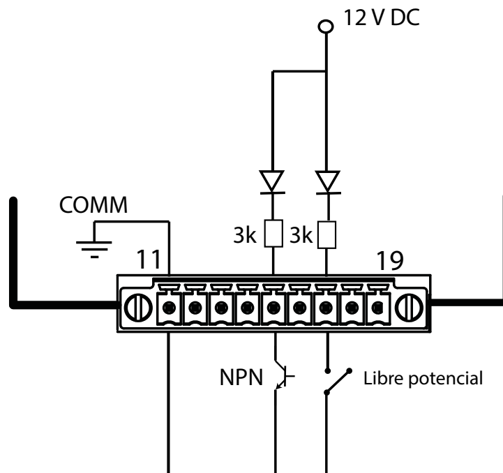
Figura 335: Esquema de conexionado, entradas digitales.
