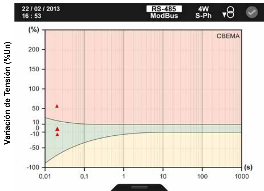
Figura 188: Curva CBEMA.
