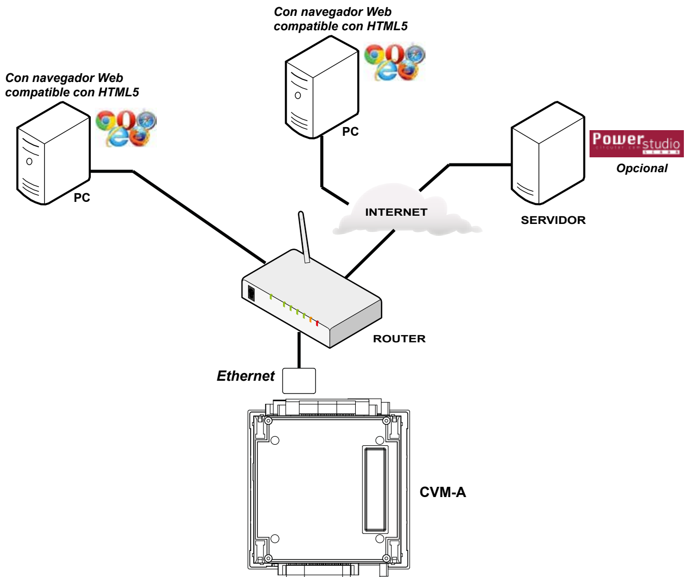
Figura 32: Esquema de conexión, Datalogger.
