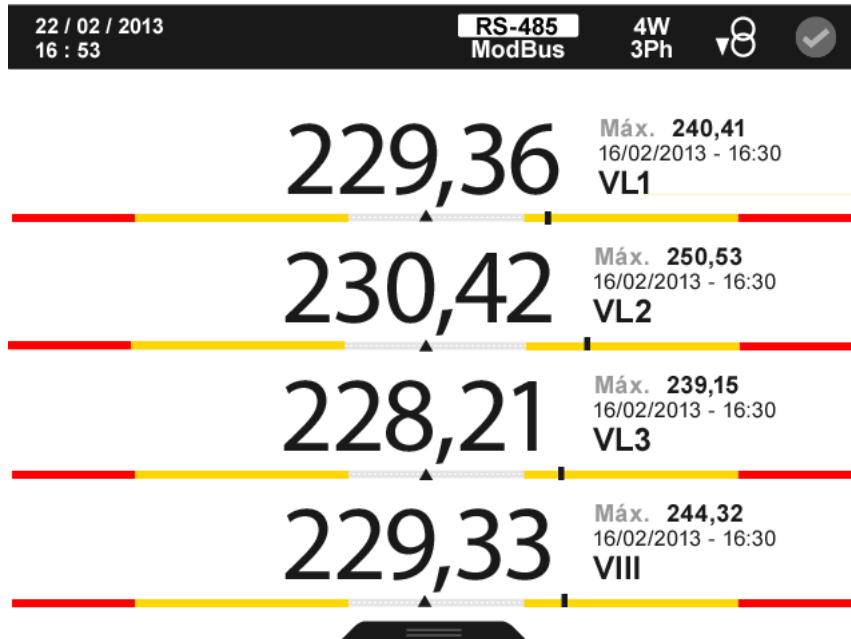
Figura 116: Parámetros instantáneos (visualizar 4 parámetros).
