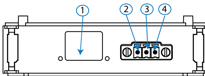
Figura 356: Bornes Módulo de comunicaciones Modbus TCP (Bridge)
