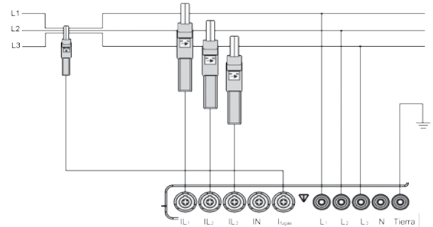
Sistema trifásico sin neutro
