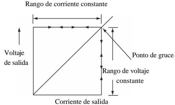
Figura 7. Voltaje constante/Corriente constante características
