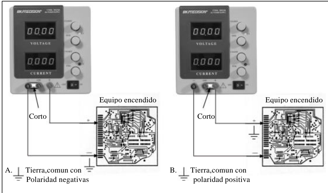
Figura A y B .Posibilidades de conexiones etierra
