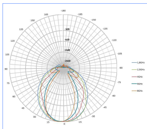
Patrón vertical Línea HyperLOG 30 X
