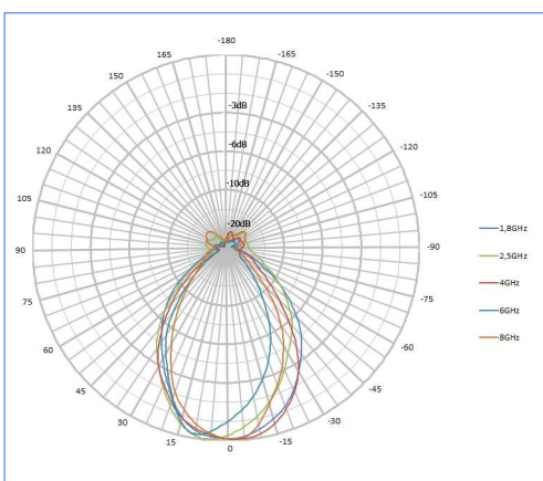
Patrón horizontal Línea HyperLOG 30 X
