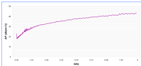
Factor de antena HyperLOG 3080
