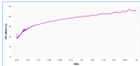
Factor de antena HyperLOG 30100
