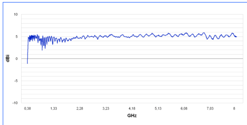
Diagrama de ganancia HyperLOG 3080
