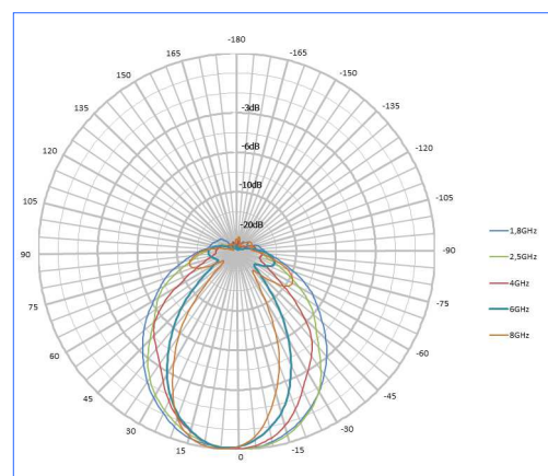
Patrón vertical Línea HyperLOG 30xx
