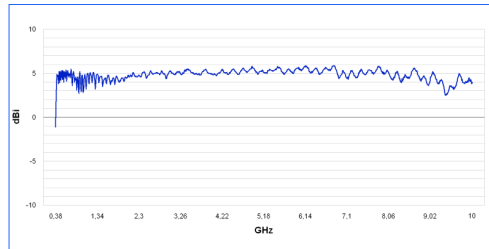
Diagrama de ganancia HyperLOG 30100
